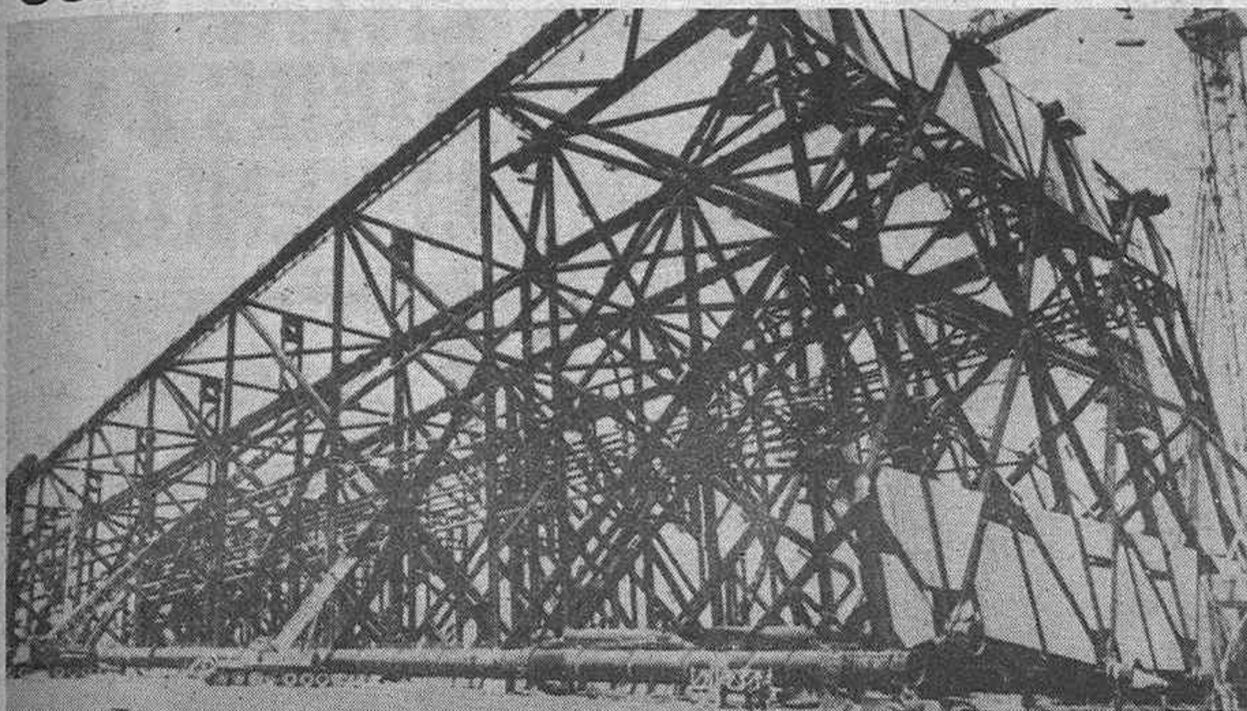
Estructura fija para la prospección petrolífera que va destinada al campo petrolífero denominado «Campo Casablanca», localizado en el mar Mediterráneo a unos 50 kilómetros al sur de Tarragona.
