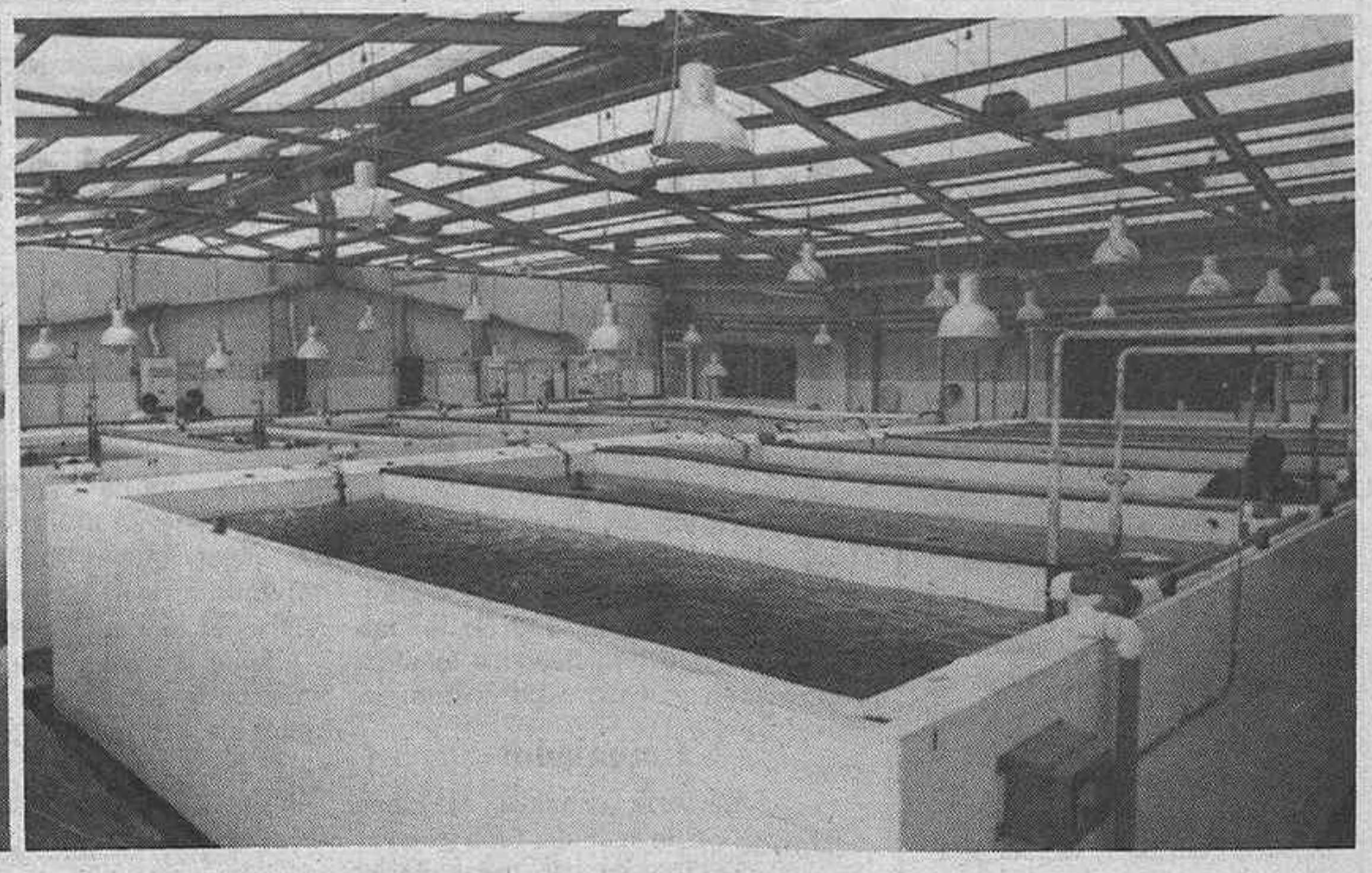
Tanques de 2.500 litros de capacidad donde los reproductores efectúan las puestas. Se utilizan también para la cría de larvas. Vista general de los tanques de 12.000 litros para mantenimiento de reproductores y cría de larvas y alevines.
