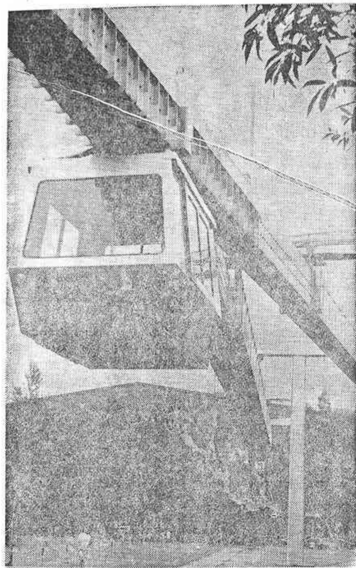
En un túnel experimental de 180 metros de longitud construido en Düsseldorf, se han iniciado las pruebas prácticas de un nuevo medio de transporte para servicios de cercanías...
