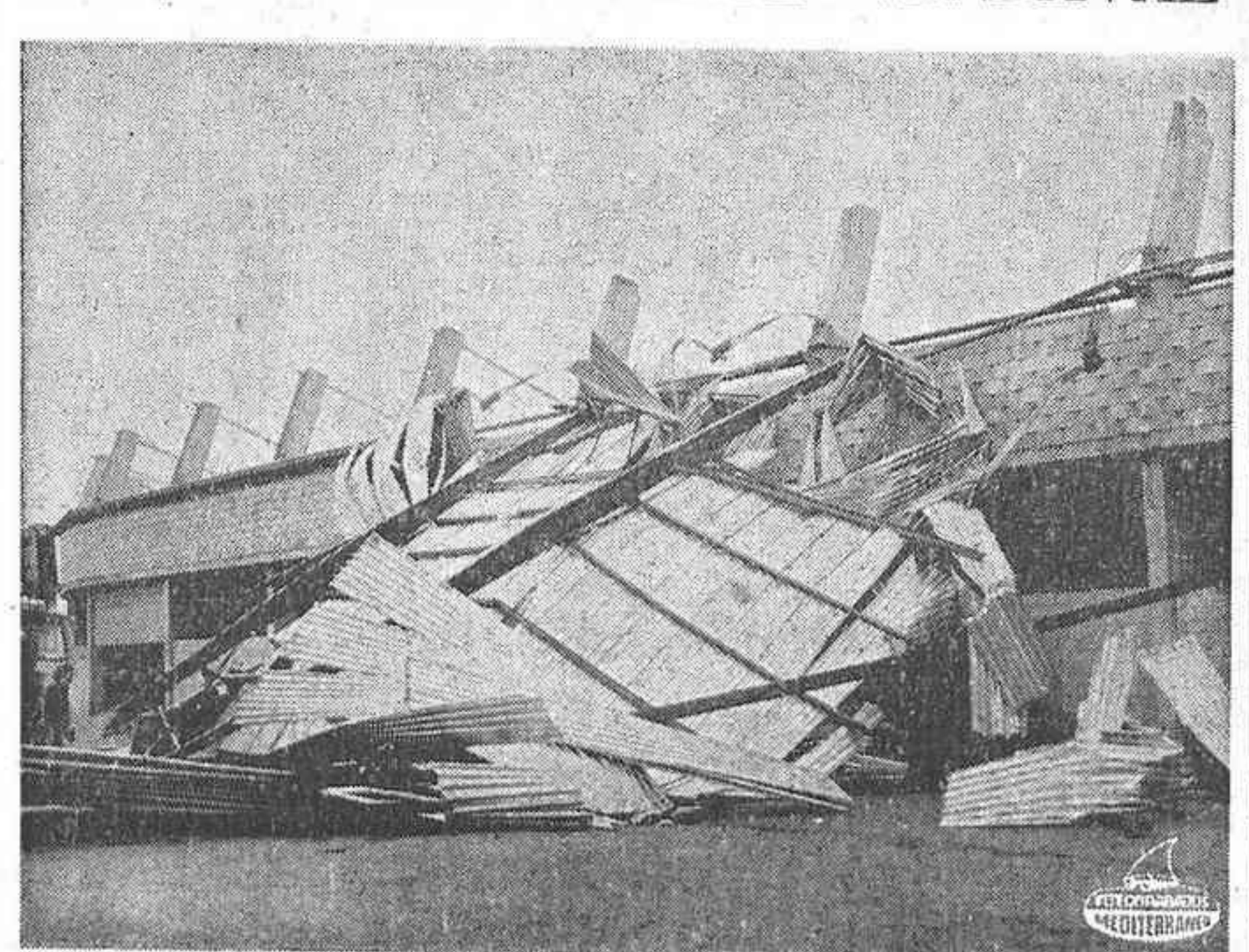
SALAMANCA. — Unos 700 metros cuadrados de cubierta del estadio Helminático se hundieron a causa del fuerte vendaval que azotó la provincia de Salamanca. Por fortuna el estadio estaba vacío y no hubo que lamentar víctimas. FOTO CIFRA GRAFICA.
