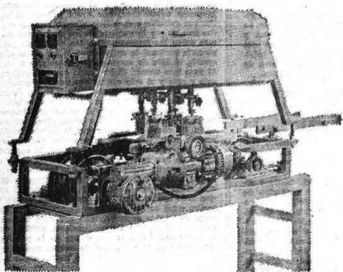
PINCELADORA AUTOMÁTICA PARA AZULEJOS EN MARCIA CON ESMALTE FRESCO, VERTICALMENTE OSCILANTE MODELO 701
