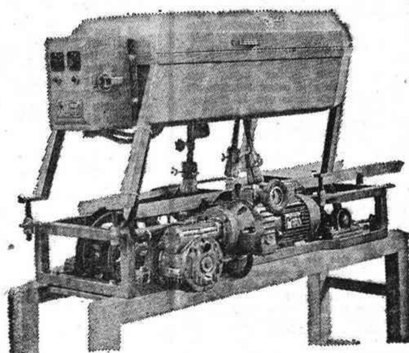
PINCELADORA AUTOMÁTICA PARA AZULEJOS EN MARCIA CON ESMALTE FRESCO, TRANSVERSALMENTE OSCILANTE MODELO 711
