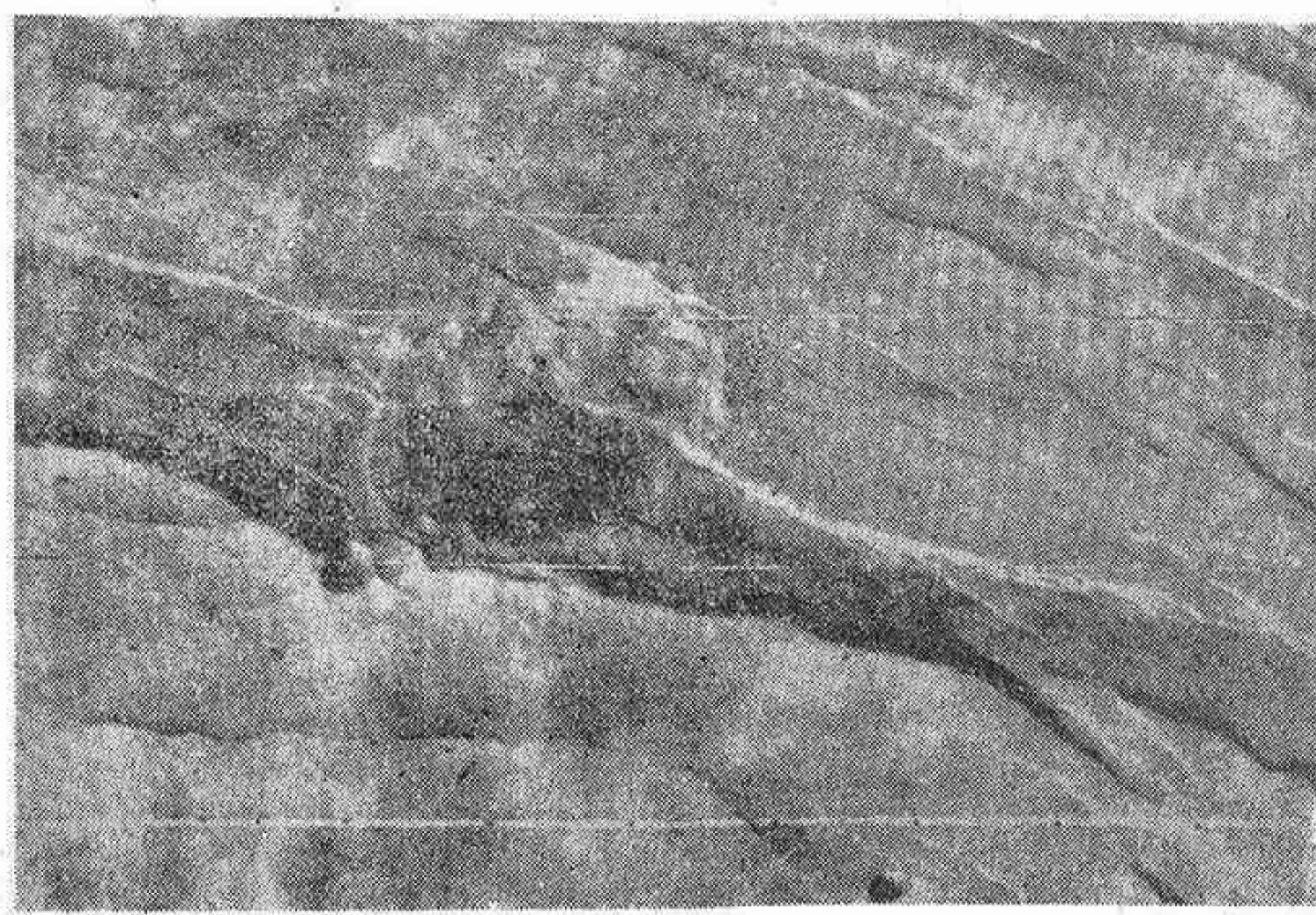
PASADENA (California).—El «Vikingo II» ha comenzado a buscar un lugar de aterrizaje sobre Marte, con fotos de las cámaras de televisión sobre una región llamada Alba Patera o «Platillo Blanco». «Situada a unos 110° Oeste, de longitud, 44° Norte de latitud, la región es una baja planicie volcánica». Las fallas sobre la corteza cortan la planicie, según puede apreciarse en esta foto, facilitada por la NASA. Tomada durante las mañanas marcianas con el sol muy elevado y con nubes atmosféricas, esta foto muestra una superficie que, aparentemente, es suave. La foto fue captada desde unos 2.200 kilómetros y muestra una extensión de unos 6.500 kilómetros cuadrados. El «Vikingo II» aterrizará a comienzos de septiembre.— (Telefoto Cifra Gráfica-Upi)
