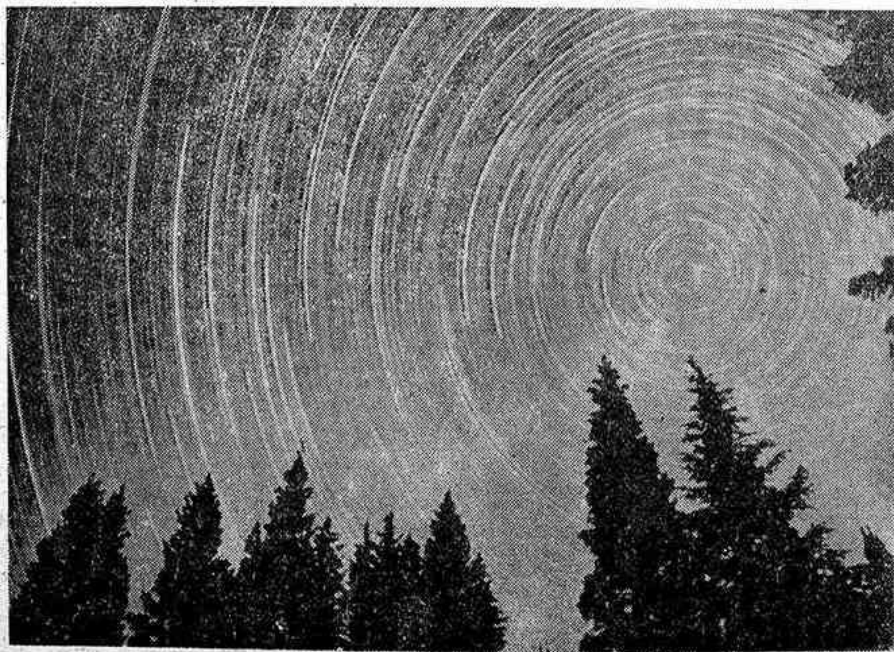
CRESTED BUTTE (Colorado).—Esta fotografía, tomada con tres horas de exposición, da la sensación de que las estrellas están moviéndose sobre la Tierra. En realidad la causa de esta imagen es la rotación de la Tierra. El centro de los círculos es la estrella Polar, la estrella del Norte. (Telefoto Cifra Gráfica)
