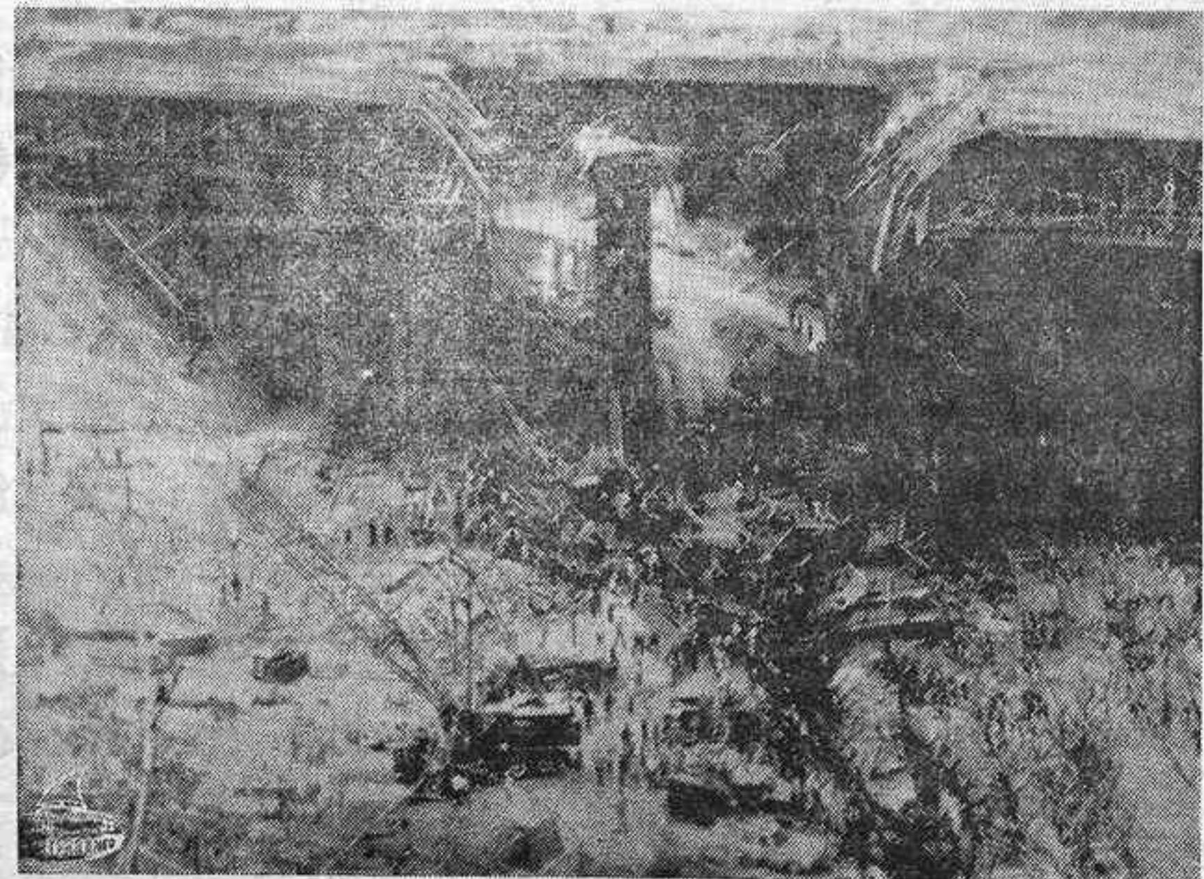
PASADENA (California). — Una parte de la «Foothill Freeway» (autopista) ha caído sobre Arroyo Seco, después de derrumbarse el martes, resultando muertas unas cuatro personas, todas ellas obreros. Grupos de búsqueda y salvamento buscan a los supervivientes entre las ruinas. Otras diez personas resultaron heridas. — (Telefoto CIFRA GRAFICA-UPI)
