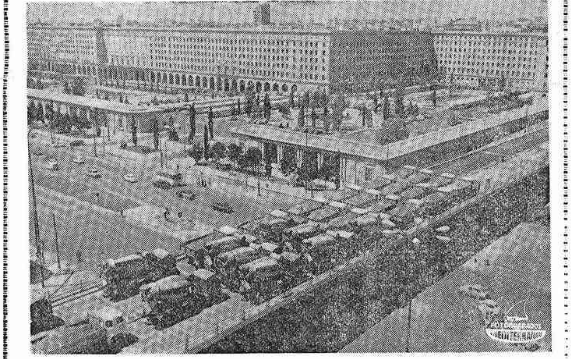
Con los camiones cargados que suponían mil toneladas de peso, ha sido realizada la prueba de carga del paso elevado construido sobre la confluencia del Paso de la Castellana y la Avenida del Generalísimo en Madrid, que une directamente las calles de Joaquín Costa y Raimundo Fernández Villaverde. Con aparatos especiales se comprobó la resistencia del puente y su flexibilidad. En la foto vemos un momento de la prueba. — (Foto F.I.L.)
