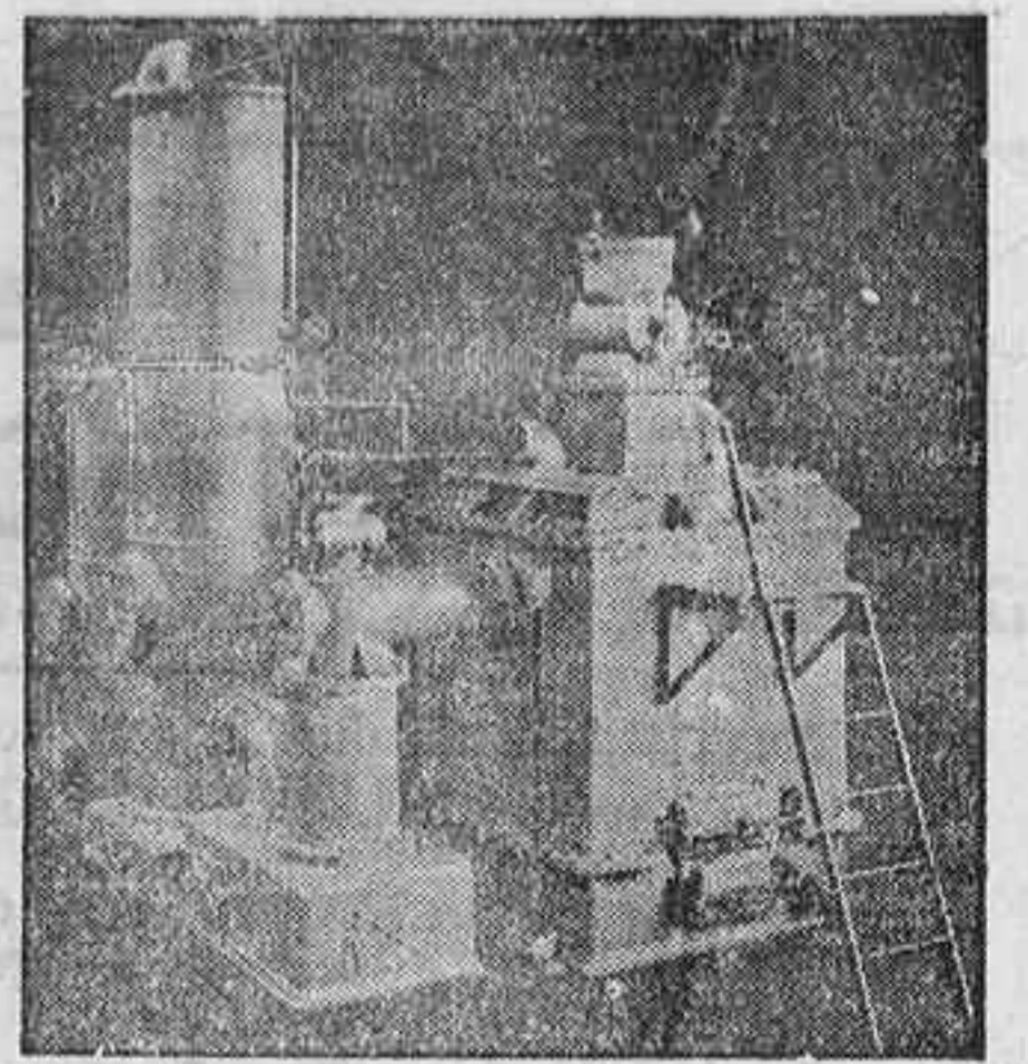
Gasógeno sencillo
