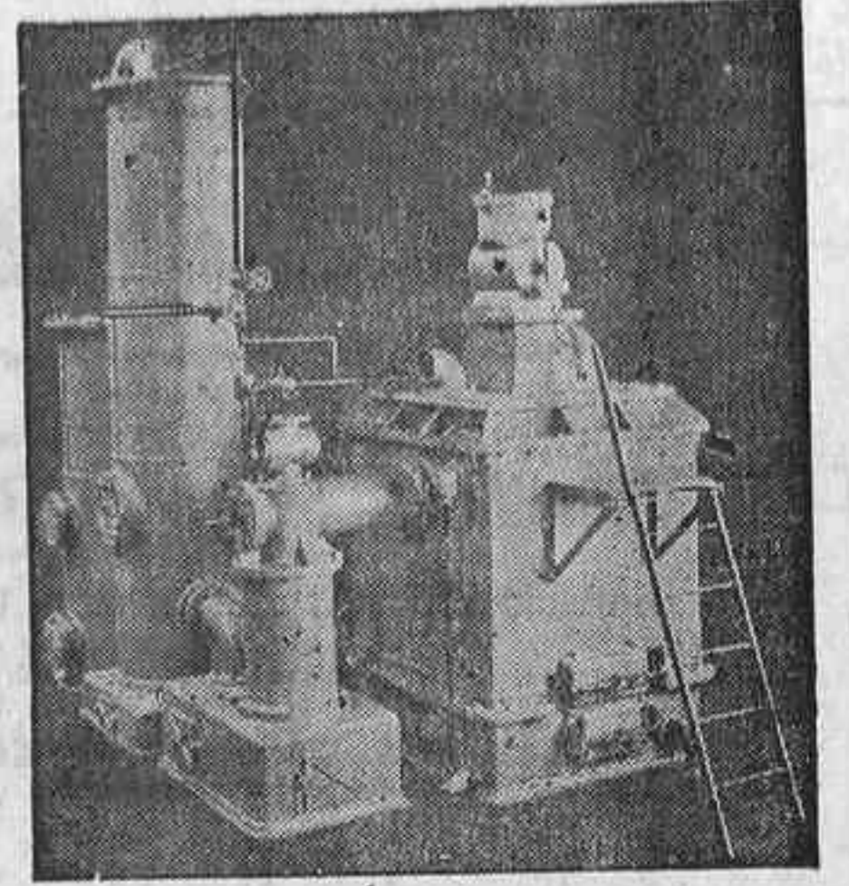
Gasógeno sencillo
