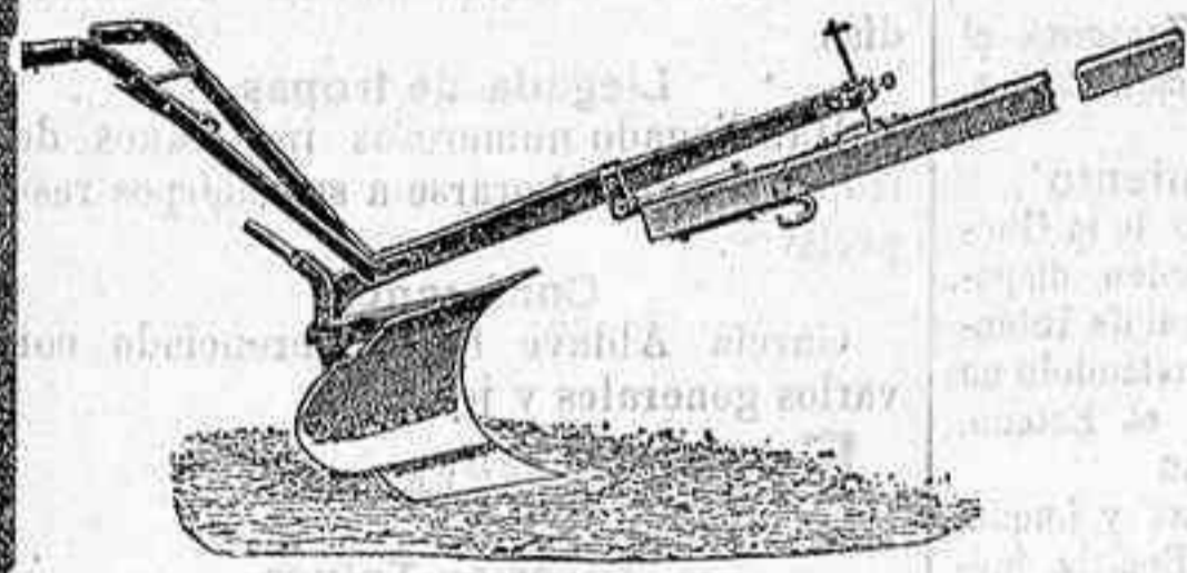
Arado Janus K. S. 1-tipo R. S. N. 5
