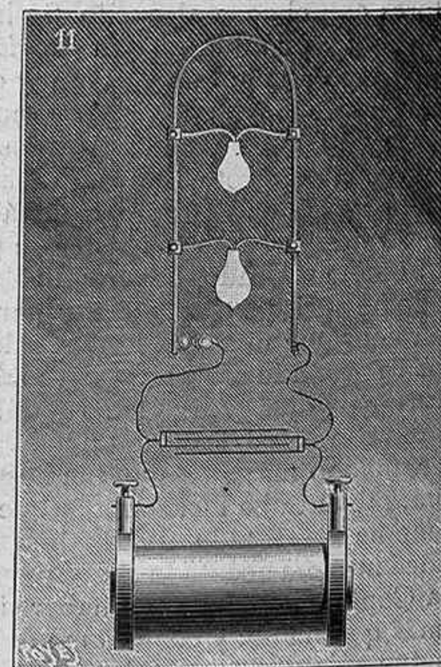
Fig. 11. Experimentos de M. Tesla. - Iluminación de lámparas de incandescencia provistas de shunt mediante un conductor de cobre de bastante diámetro. Producción de nudos y abultamientos en el conductor.
