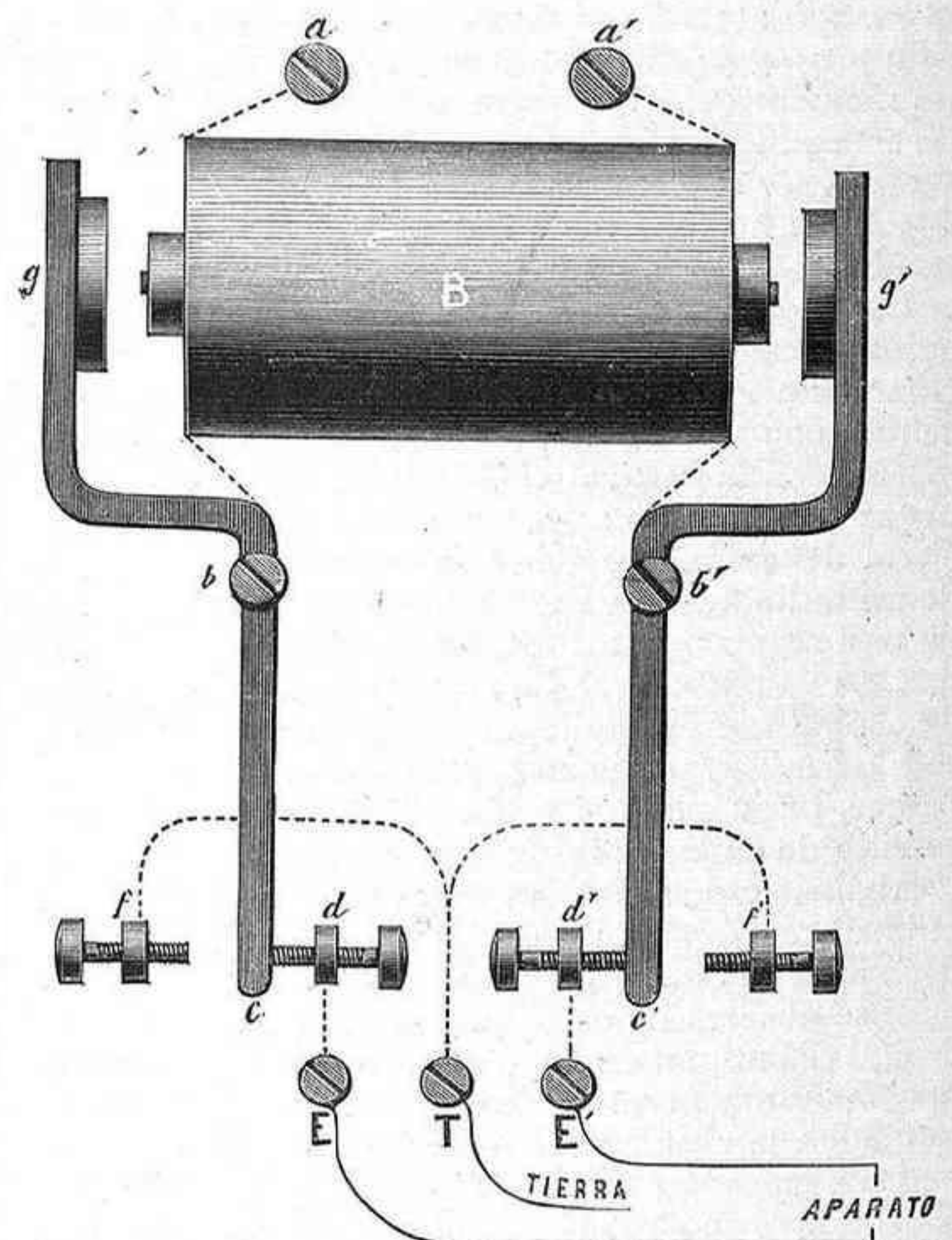
Pararrayos Ferrer para líneas eléctricas
