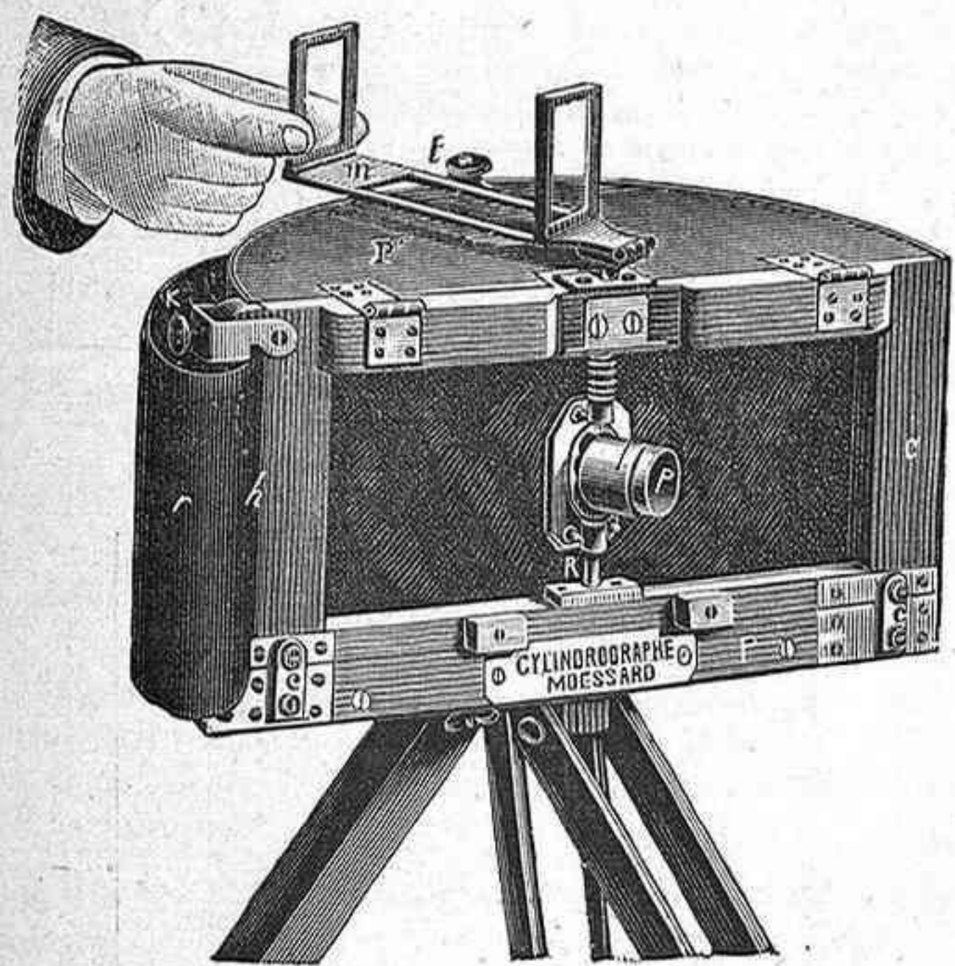
Fig. 1. El cilindrógrafo
