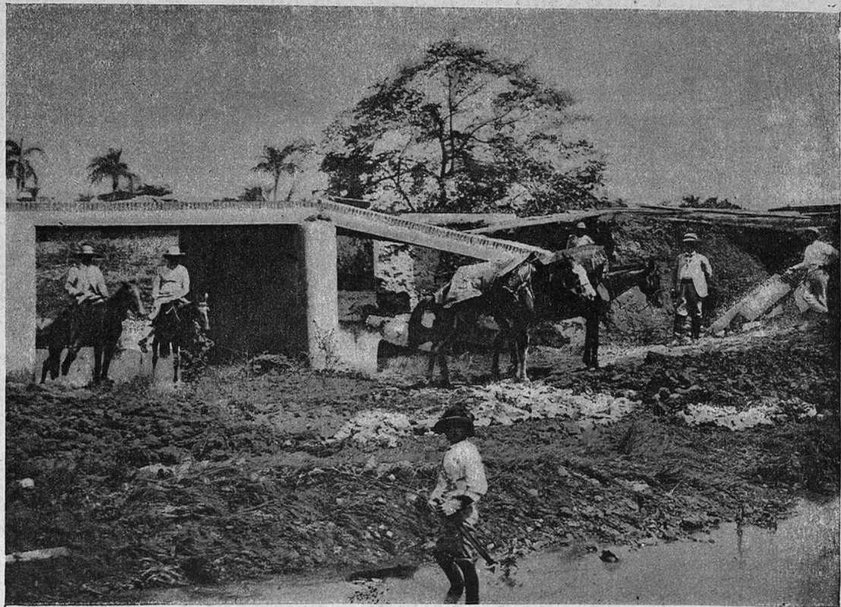
ISLA DE CUBA.—DESTROZOS CAUSADOS POR LA INUNDACIÓN DEL 2 DE OCTUBRE ÚLTIMO EN LA CARRETERA GENERAL DE VUELTA ABAJO.
