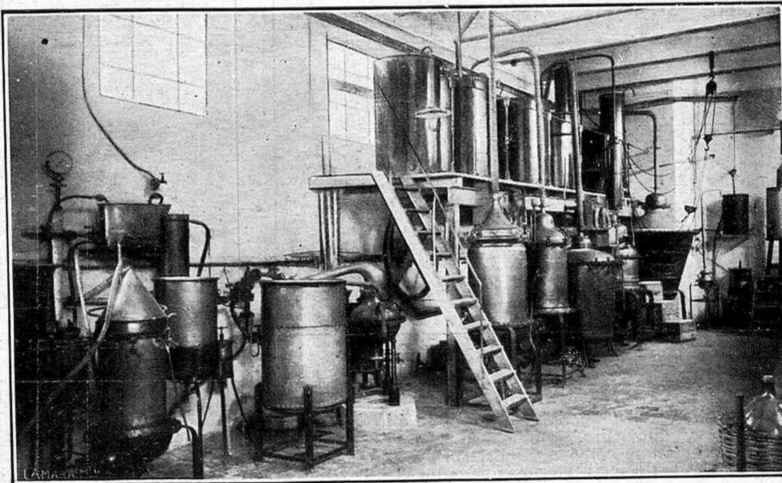
Un aspecto de la sala de aparatos de destilación
