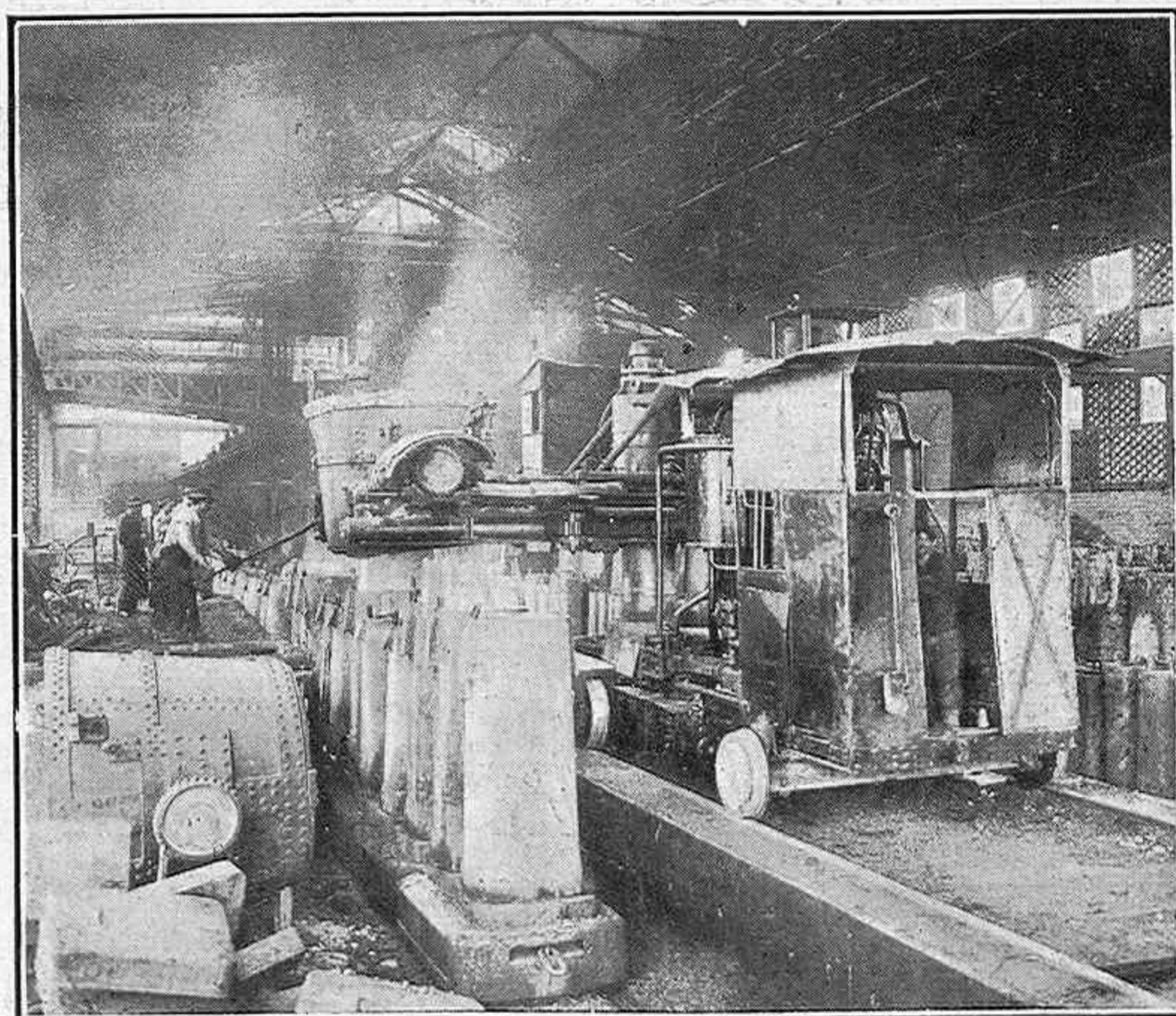
Producción de acero Thomas en los altos hornos de Auboné
