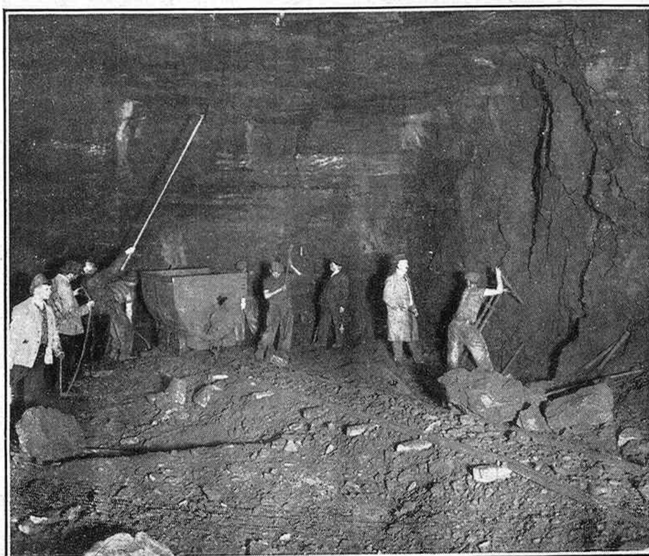
Un frente de arranque en la mina de Auboné (Lorena)
