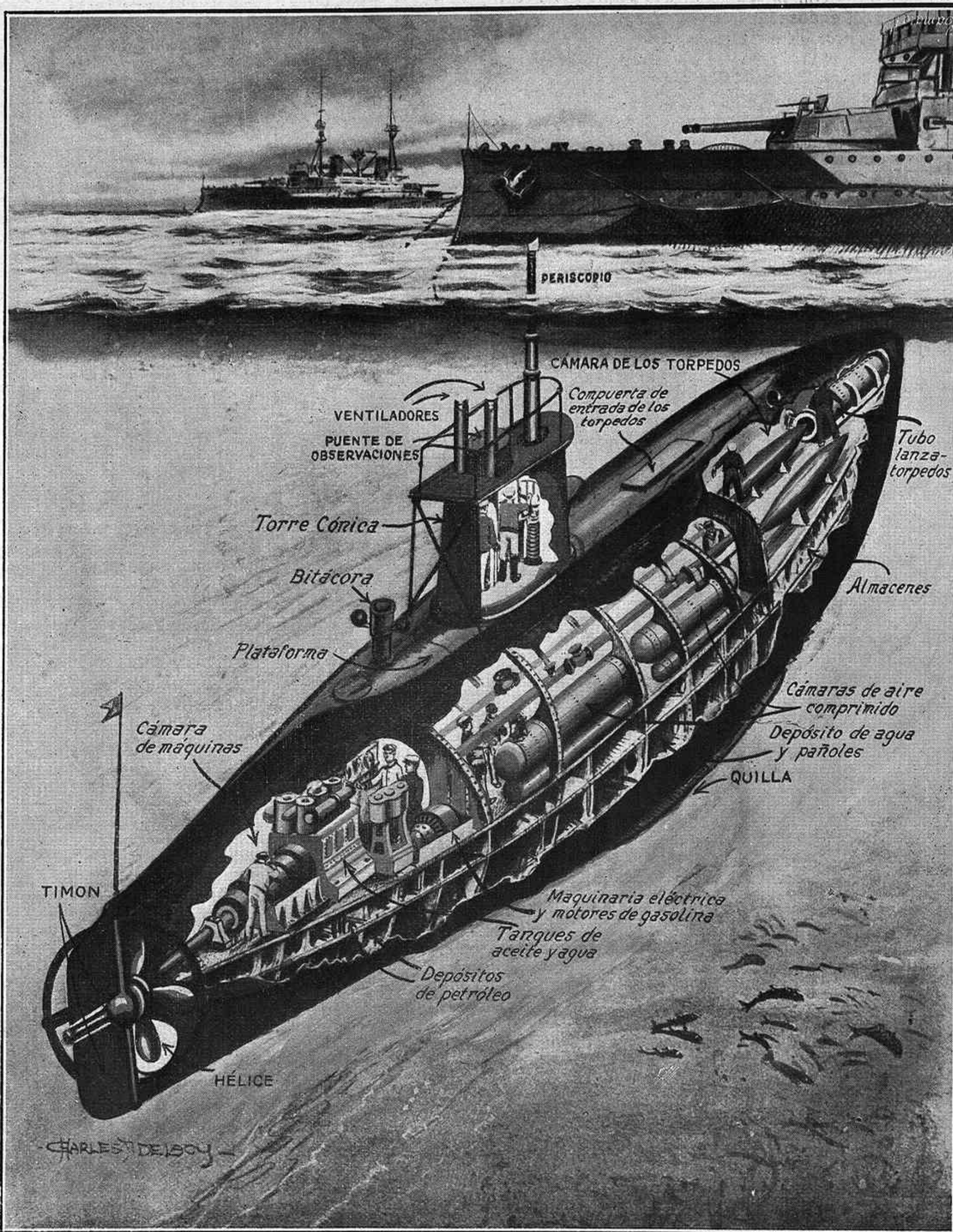
El grabado adjunto representa el submarino inglés A-7, uno de los varios buques sumergibles que ha perdido la poderosa escuadra de la Gran Bretaña. Data este barco de Abril de 1904 y fué botado al agua el mismo día que el A-8. De la serie A, eran 13 los submarinos construidos por la soberbia Albión, y para dar razón á los supersticiosos, se han hundido ya en las aguas, para siempre, cinco de estos buques: el A-1, el A-3, el A-5, el A-7 y el A-8. De otros tipos ha perdido Inglaterra el C-11, el E-5, y el C-14. Los primitivos tipos de submarinos, como el A-7, sólo los empleaba la Gran Bretaña para instrucción y defensa de costas
