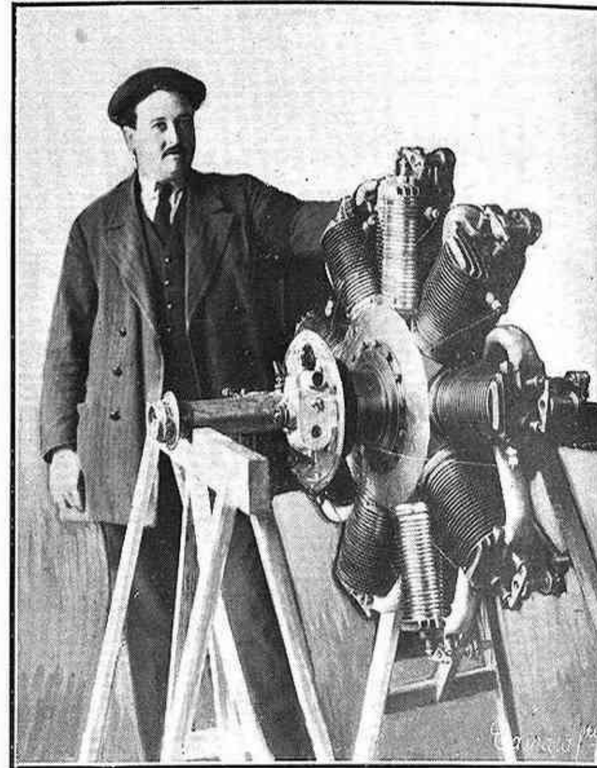
Motor á esencia, de 80 caballos, que constituye la última palabra de la Mecánica en la generación de fuerza con pequeño volumen
