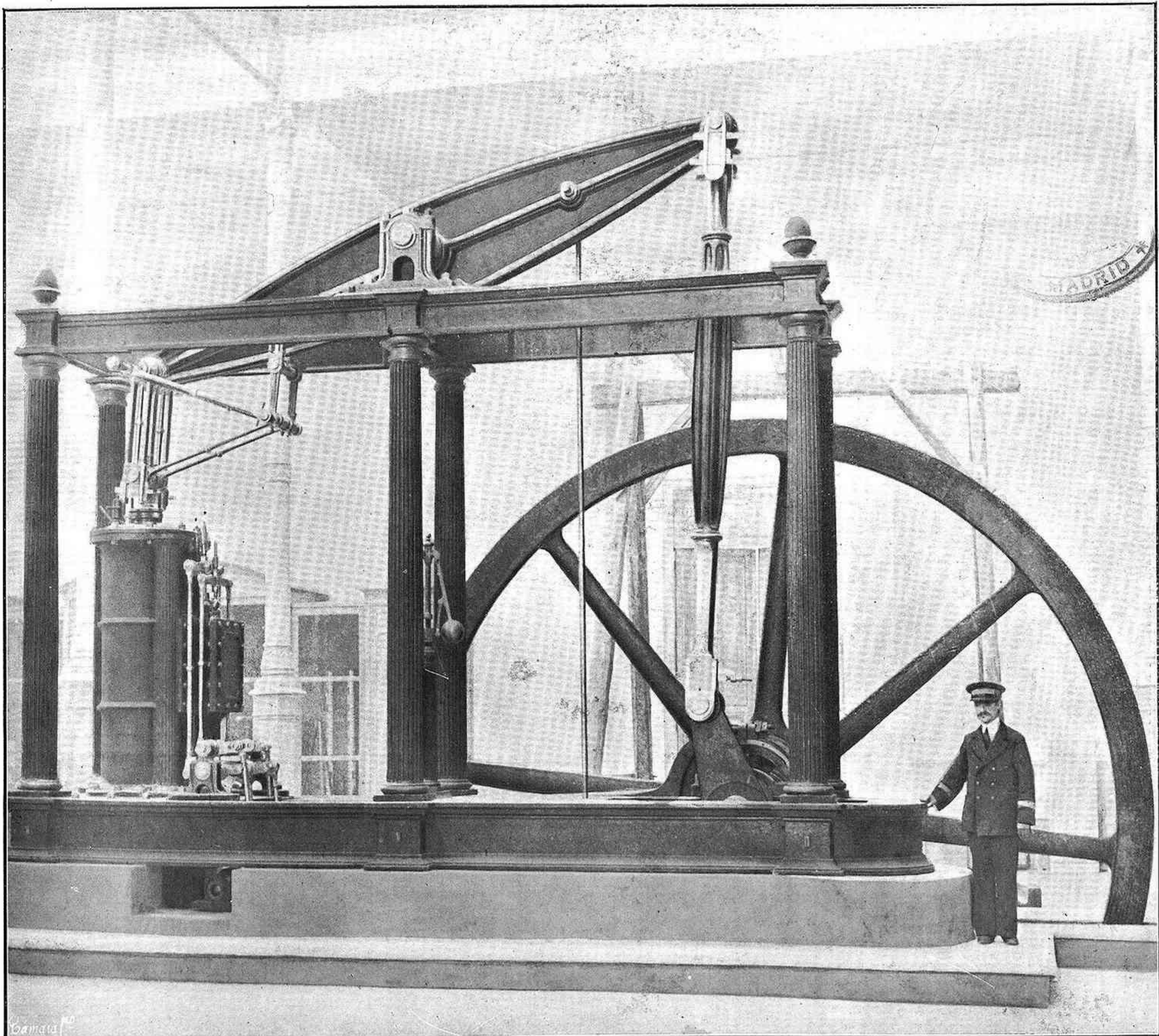
Máquina de vapor de 25 caballos, sistema Watt, primera de sus condiciones importada á España y que ha sido instalada como curiosidad histórica en la Escuela de Ingenieros Industriales
