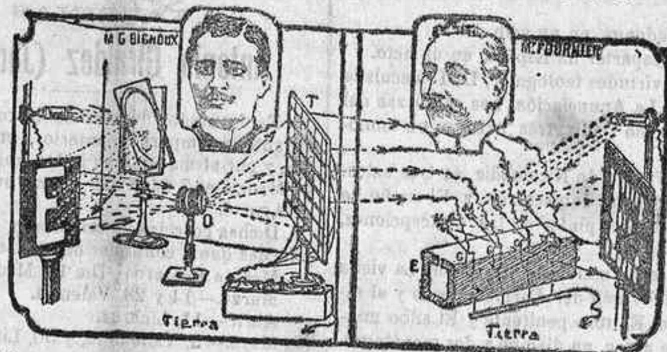
O. Objetivo.—T. Cuadro de células de selenio.—M. M. Espejos.—G. Galvanómetro.—C. Electroimanz.
