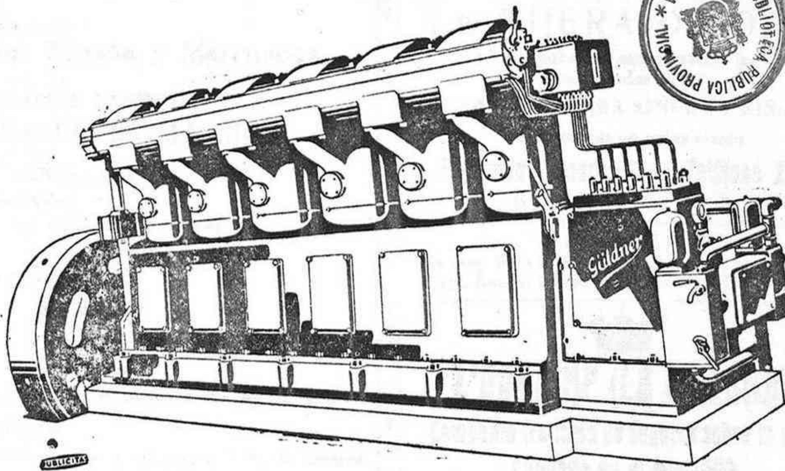
Motores Diesel «Güldner» hasta 1.200 caballos
