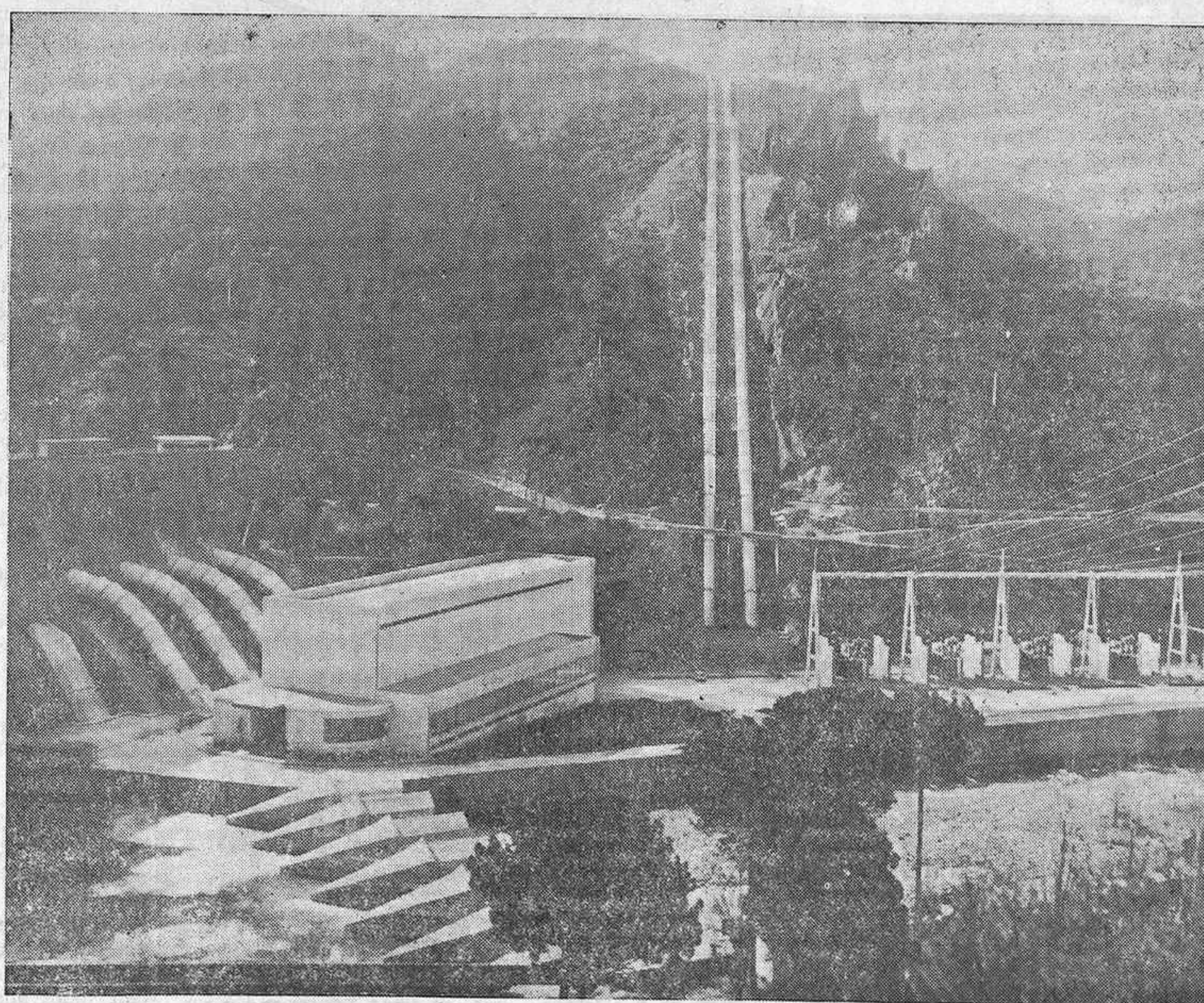
CENTRAL BOLARQUE II — ARRANQUE DEL TRASVASE TAJO - SEGURA
