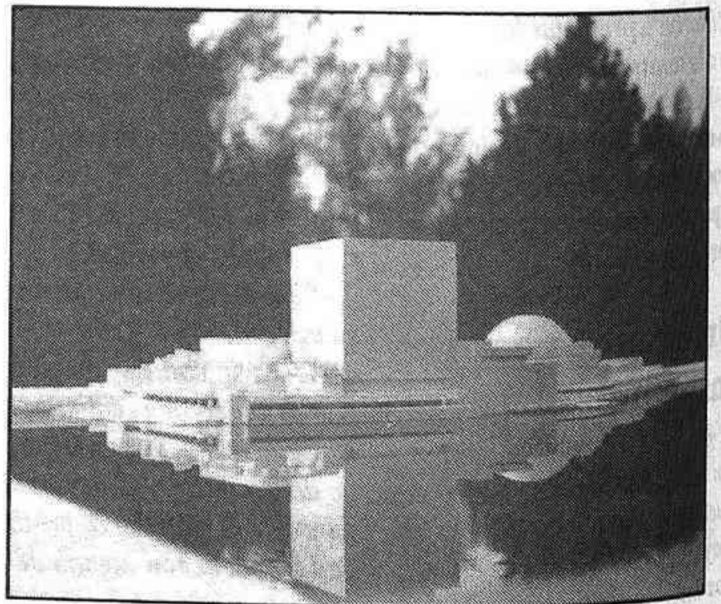
Maqueta del pabellón de España en la Expo '92
