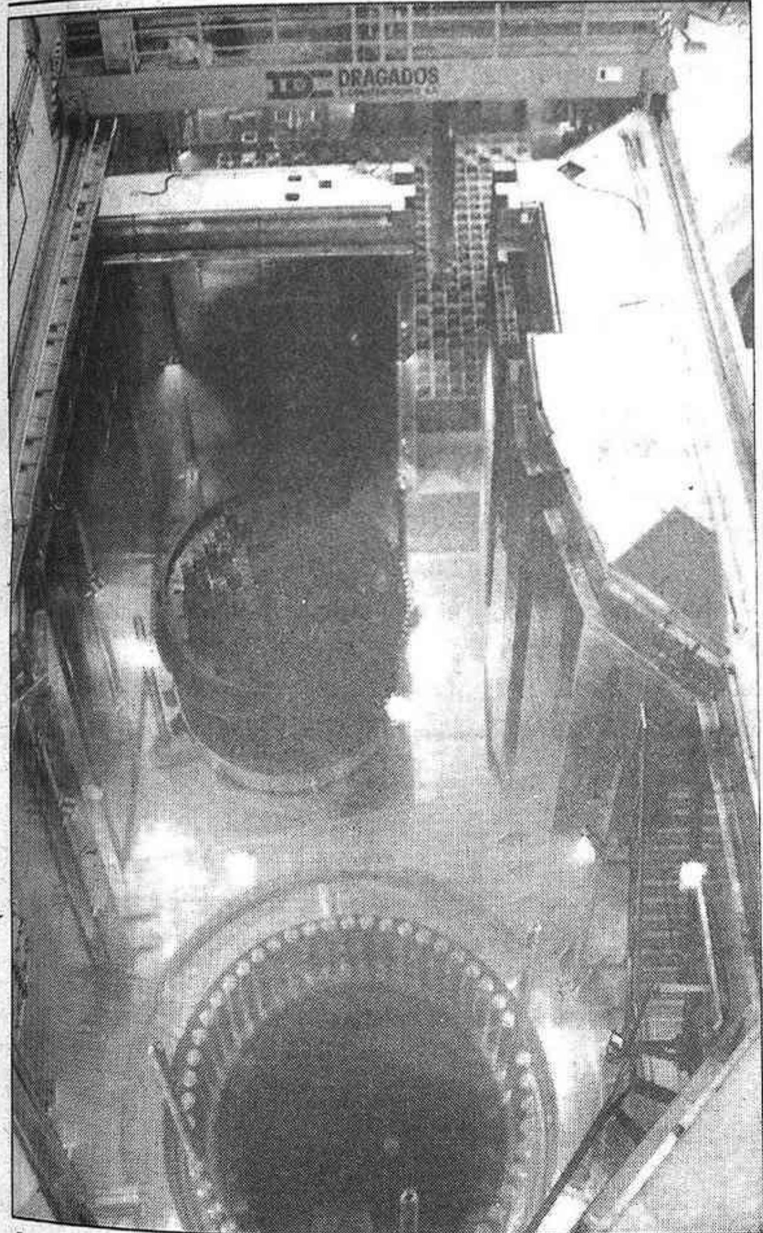
Apertura de la vasija del reactor para proceder a una recarga de combustible en Trillo I
