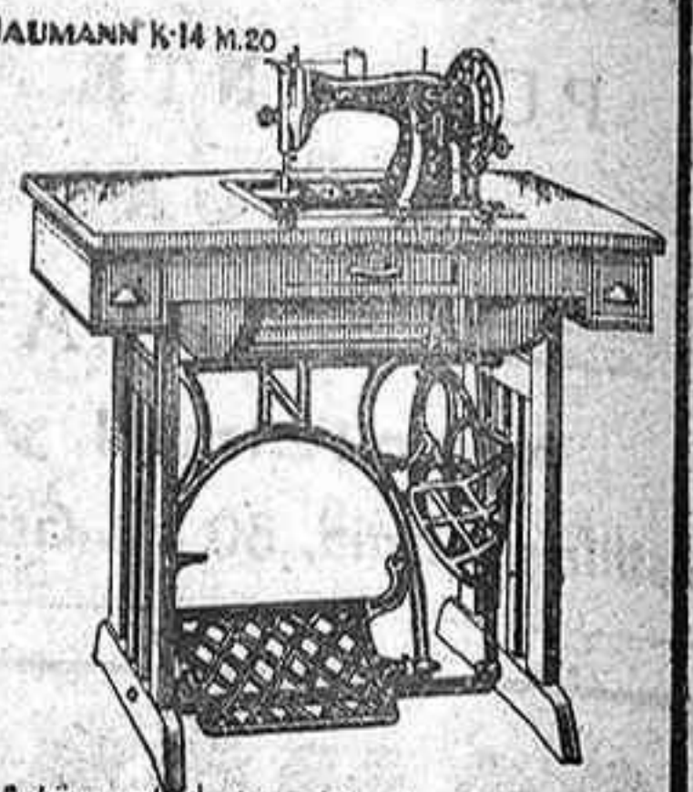
NAUMANN K-14 M.20 Bobina central, Armaduta de madera, Mueble lundible, dos gavetas y cajón. Cierre persiana.
