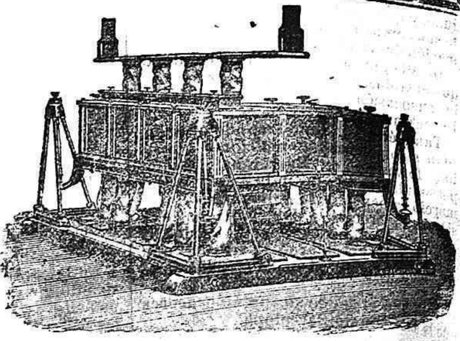
Plansichter DAVERIO construcción, 1902.
