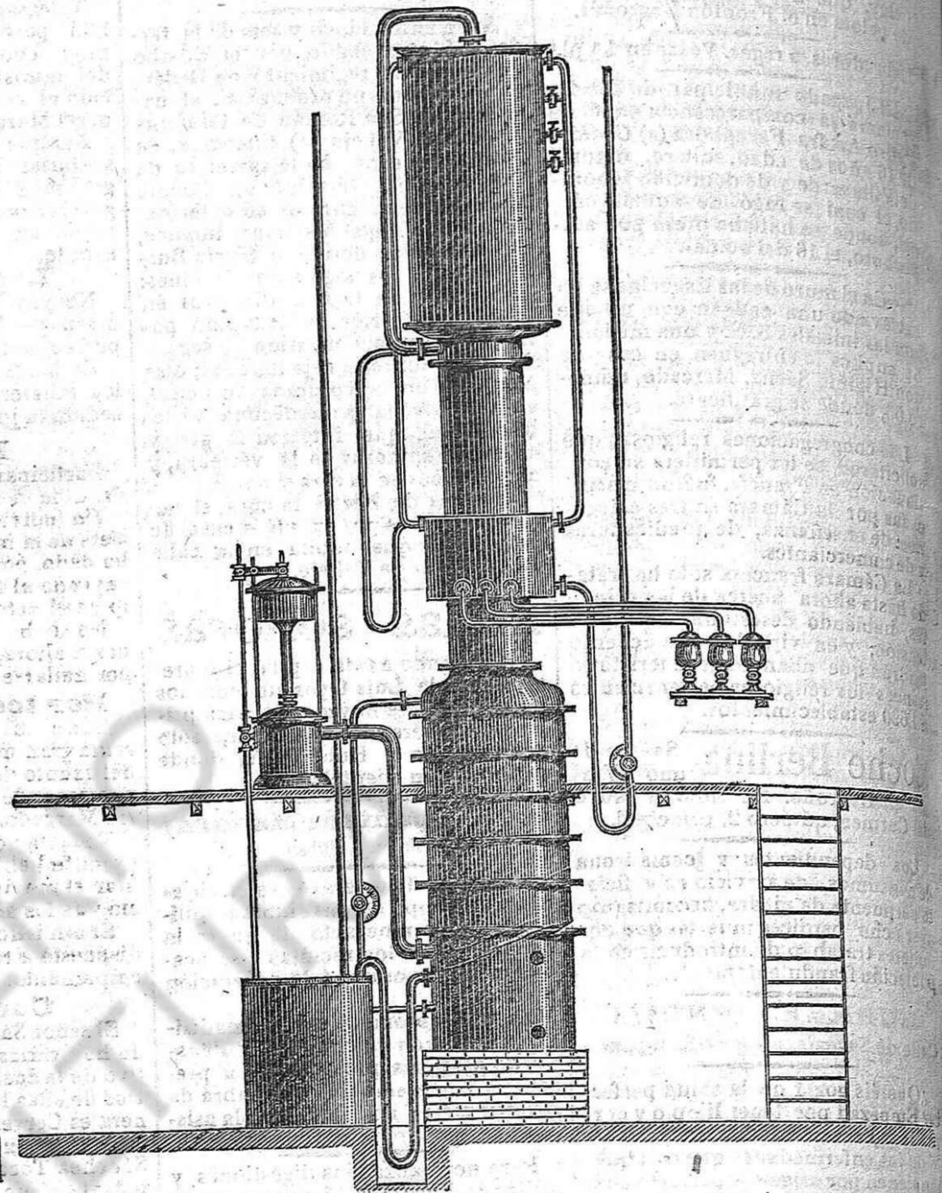
DESTILADOR DEPURADOR CONTINUO U DISCONTINUO A FUEGO DIRECTO Ó A VAPOR
