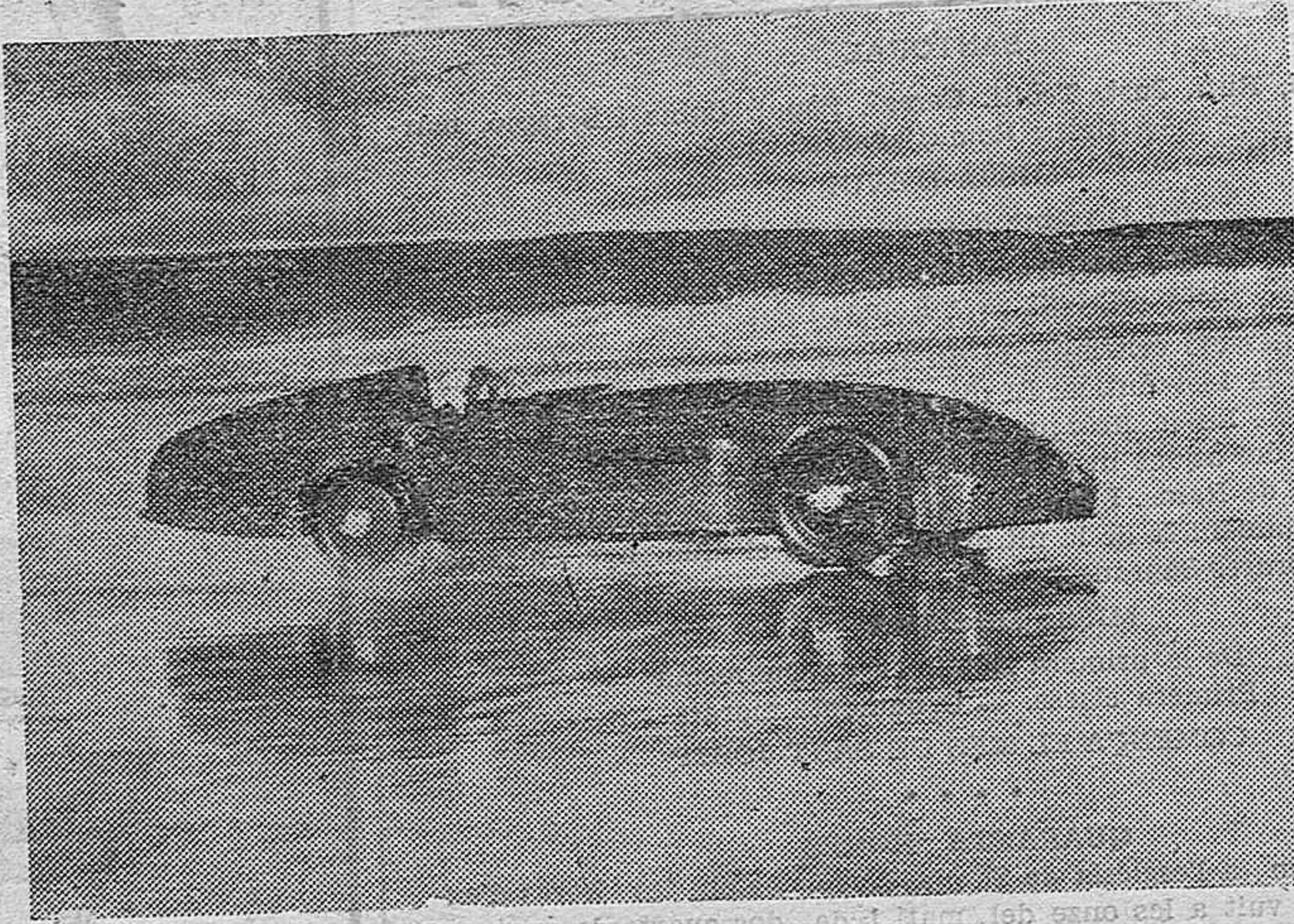
Para probar la seguridad de los motores "Diesel", para emplearlos en los aviones, el capitán Eyston, por encargo del ministro del Aire británico ha realizado pruebas de ellos con coches equipados con dichos motores, obteniendo felices pruebas. Un coche equipado con un motor "Diesel" en plena carrera. (Express-Foto)
