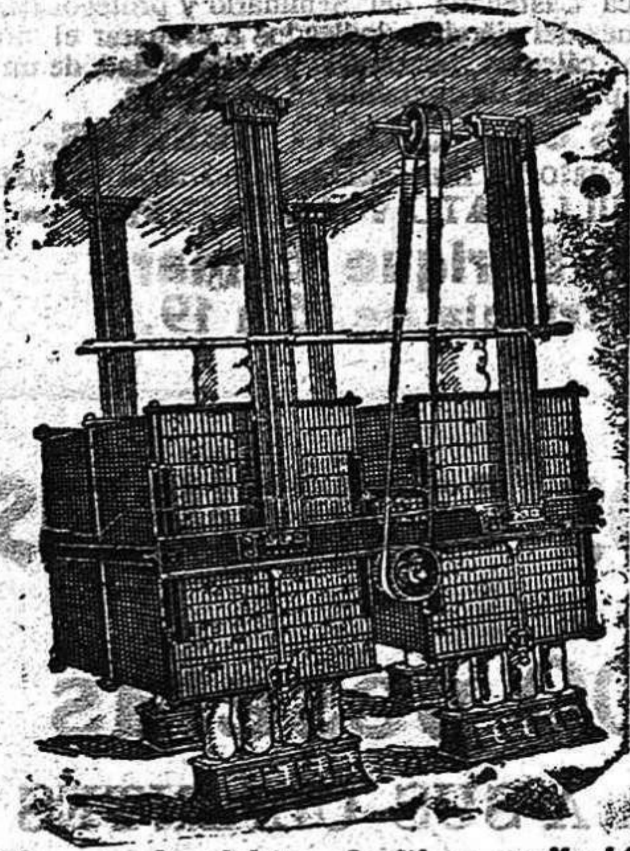
Nuevo planichter de libre oscilación y equilibrio automático.—Privilegio Buhler.
