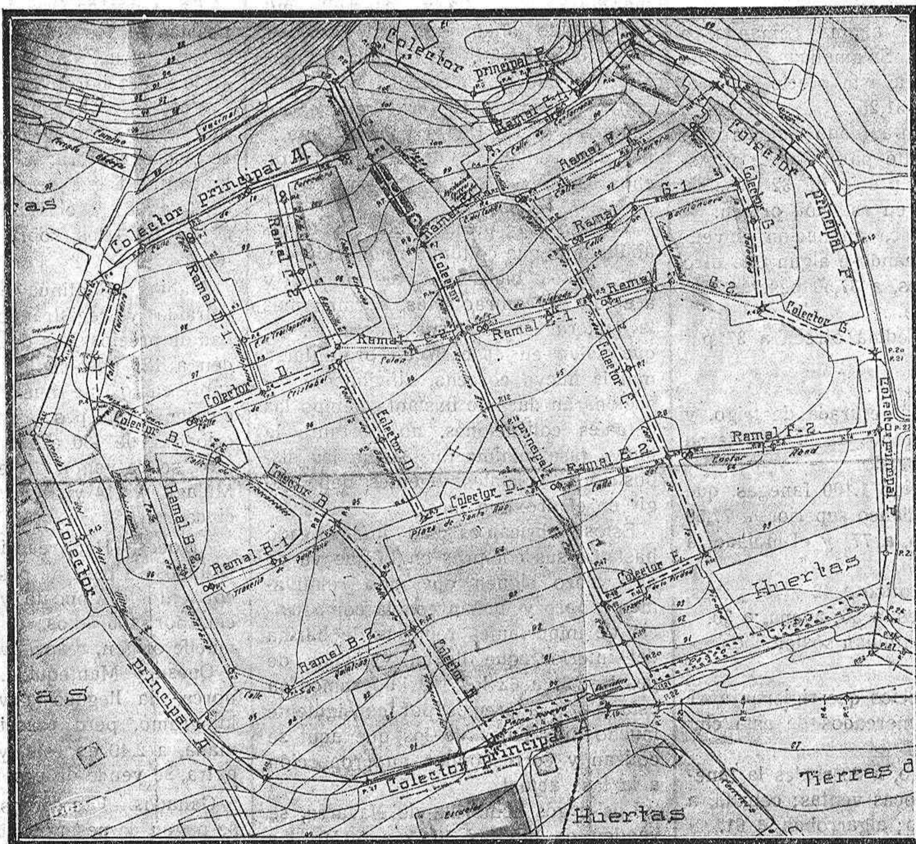
Herrera de Pisuergra.—Plano de la población, con el proyecto de alcantarillado.
