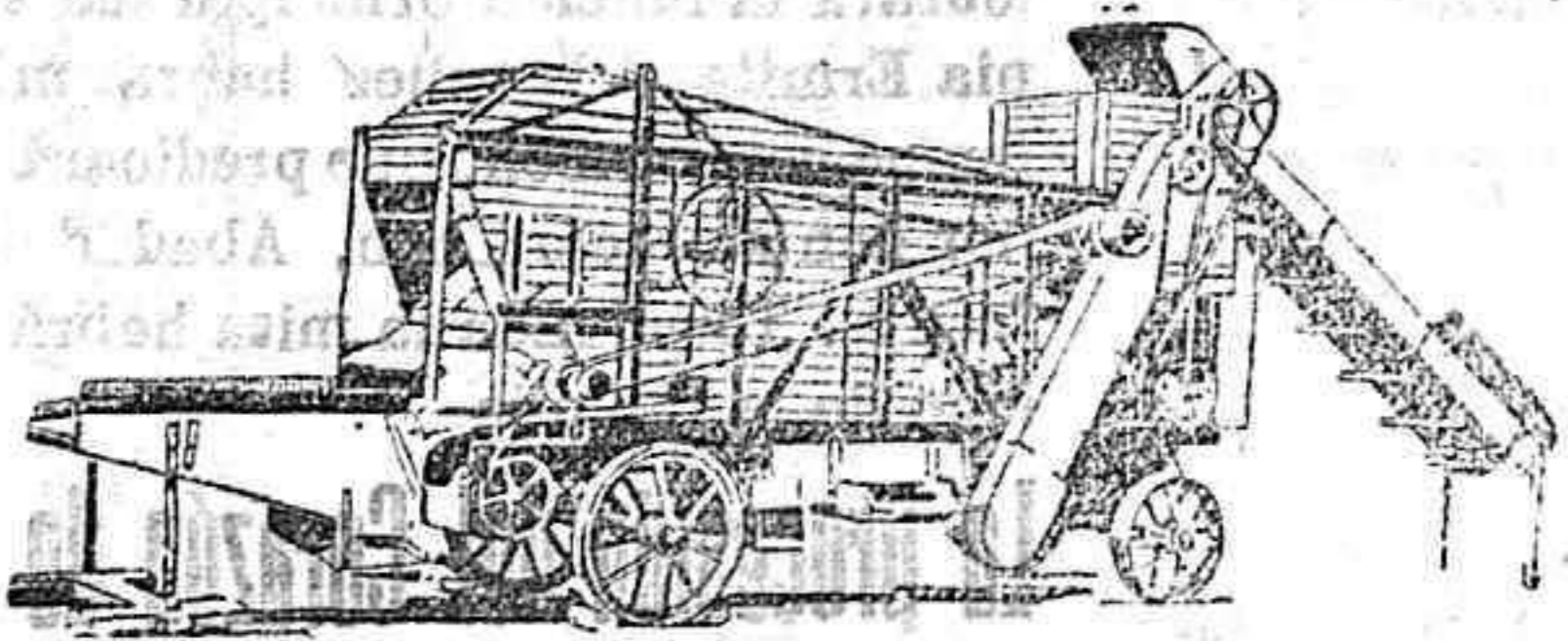
Trilladora «Triunfo Chica» con elevador de mies. Rendimiento diario de 90 a 120 fanegas de trigo diarias, según granazón.
