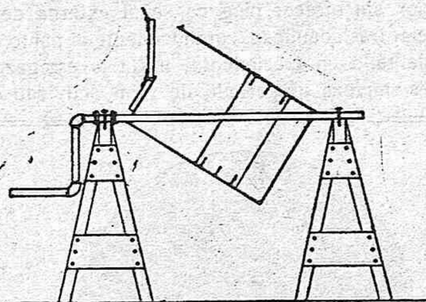
Fig. 10 Puede contruirse un rústico y económico aparato de desinfección en seco, con un bidón metálico provisto de un eje diagonal.
