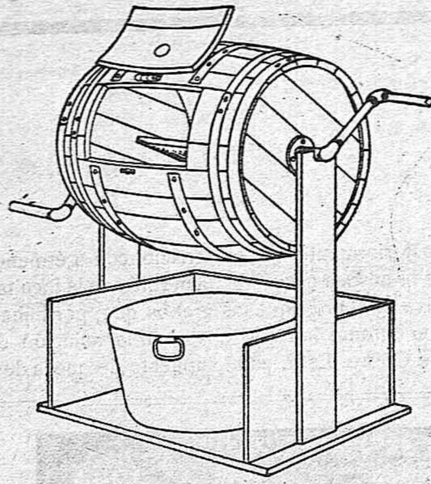
Fig. 9 Detalles del modo de adaptar el barril para desinfección en seco.
