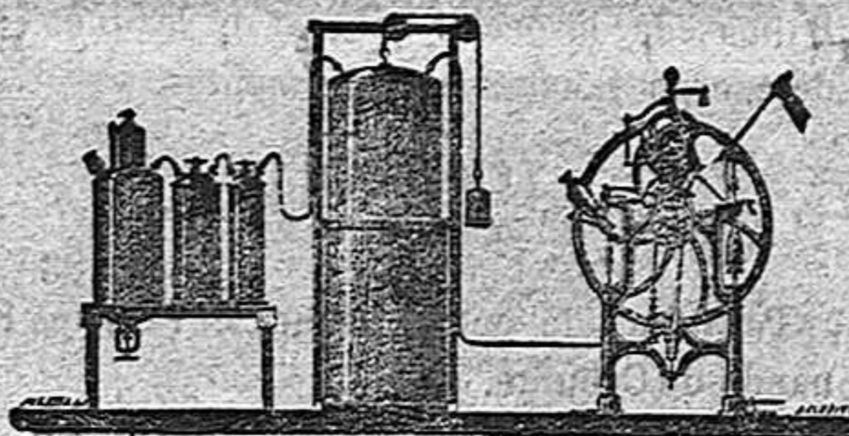
Aparatos para hacer gaseosas, Continuo con embotelladora en columnas independientes.
