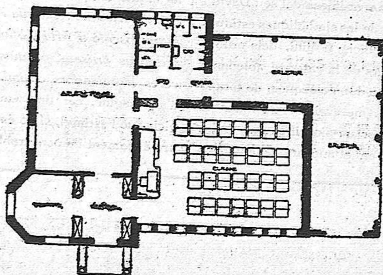
Escola de Torms. Planta
