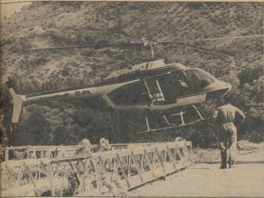
El helicóptero sobrevuela a escasa altura para poder enganchar una de las torretas. Es el primer paso de la maniobra. Luego cogerá altura y deberá situarse justamente encima del punto indicado.
