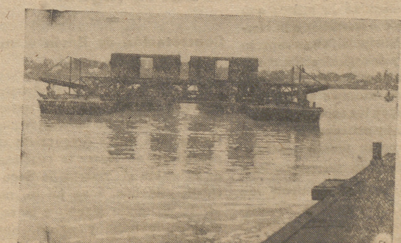
Para sustituir un puente bombardeado en Mena, Bangkok, los ingleses prepararon un transportador de barcasas para cruzar el río, y escolleras especiales para la carga y descarga. El transportador puede cargar dos vagones en cada una de las travessías
