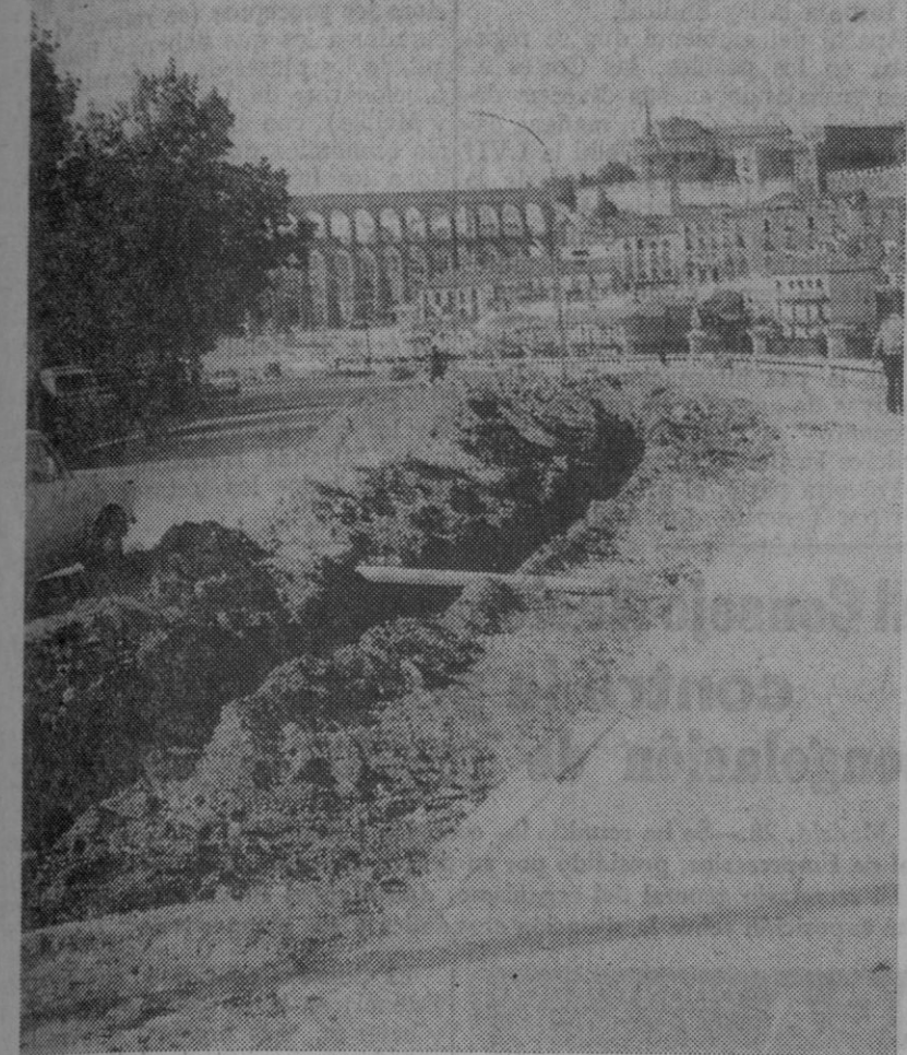
Según las obras destinadas a dejar en las debidas condiciones el aparcamiento de vehículos del P. Claret. En el grabado puede verse claramente la zanja abierta para instalación de las tuberías destinadas a cables de conducción eléctrica y a las aguas de lluvia, para impedir nuevas deformaciones en el piso del aparcamiento, que va a ser adquinado convenientemente. Y también se observa la eliminación total de árboles, a la que ya hemos hecho referencia. (Foto Antonio)
