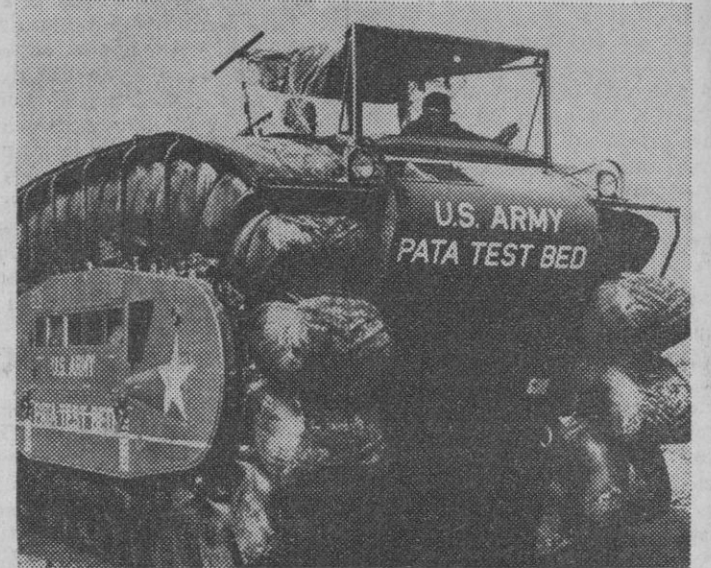
El Cuerpo de Transporte del Ejército de los Estados Unidos está perfeccionando actualmente un vehículo de carga sostenido e impulsado por cojines de aire rotativos. El nuevo tipo de transporte es conocido en inglés por la sigla "PATA" y puede llevar toneladas y cuarto de carga por toda clase de superficies acuáticas y terrestres.
