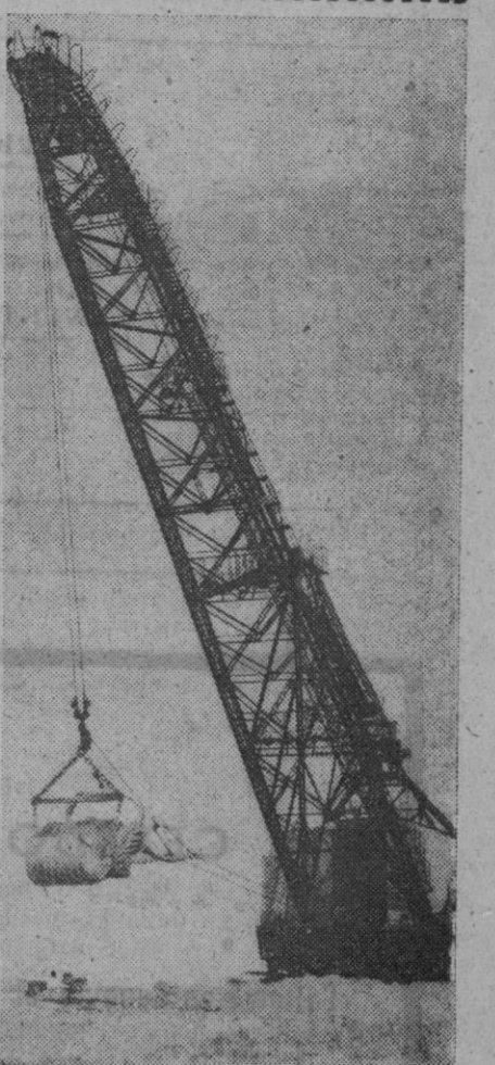
Esta gigantesca draga de arrastre es capaz de remover en una hora materiales cuyo peso sobrepase del suyo propio, mil quinientas toneladas. La máquina, que cuesta un millón y medio de libras esterlinas realiza movimientos de avance de más de dos metros y puede alcanzar un radio de más de setenta metros con un cucharón capaz de remover cincuenta y cinco toneladas de una vez.
