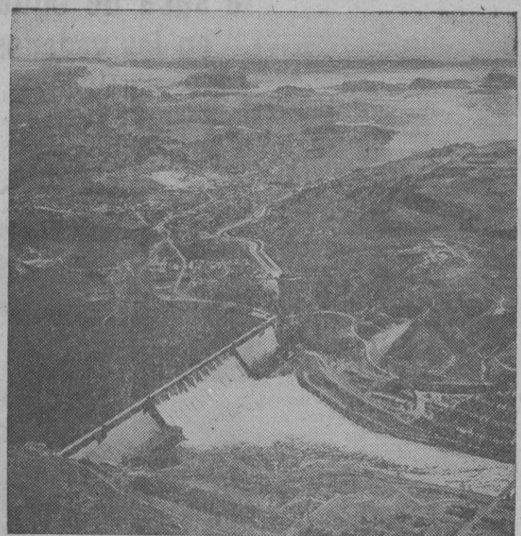
La presa Hoover, que frena las aguas del río Colorado y tiene una altura de 221 metros. Su construcción duró cuatro años. Mediante una batería de diecisiete generadores permite producir 1.354.300 kilovatios. La construcción de esta presa originó un lago artificial, el lago Mead, de 247 kilómetros de longitud y cuyas aguas benefician a siete estados.
