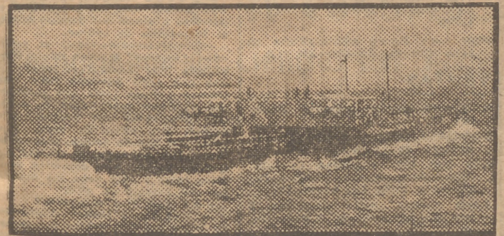
Este es el barco fluvial escocés "Lucy Ashton", durante las primeras pruebas de propulsión por reacción. Los motores van montados en el centro del barco. Las pruebas se han efectuado para calcular los efectos en la resistencia del casco en los navios con el nuevo tipo de accionamiento. (Foto A. P.)
