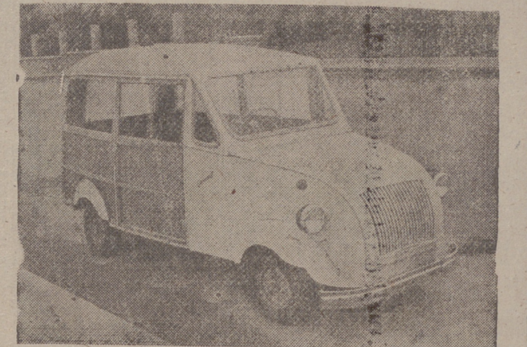
FURGONETA COMERCIAL TIPO RUBIA-BISCUTER, 2ª PLAZAS, 200 KG. CARGA.
