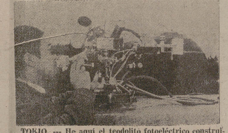
TOKIO. — He aquí el teodolito fotoeléctrico construido en el Observatorio Astronómico de esta capital para seguir la pista de los satélites artificiales lanzados por Rusia y Norteamérica. Consiste en una combinación de un telescopio, un amplificador fotoeléctrico y una pequeña cámara. Se asegura que su utilidad es superior a la de la famosa cámara Schmidt. — (Foto Torremocha).
