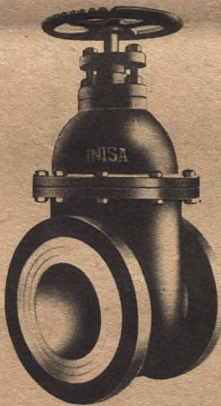
MODELO STANDARD Paso nominal mm. 40 a 1.000 Presión trabajo Hasta 16 Kgs. cm. 2
