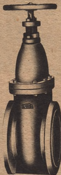
MODELO DIN Paso nominal mm. 40 a 500 Presión trabajo Hasta 25 Kgs. cm. 2
