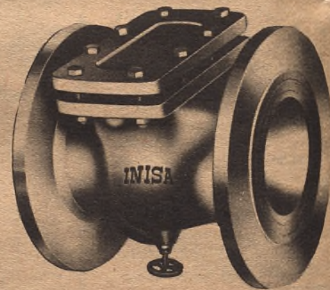
MODELO STANDARD Paso nominal mm. 60 a 800 Presión trabajo Hasta 16 Kgs. cm. 2
