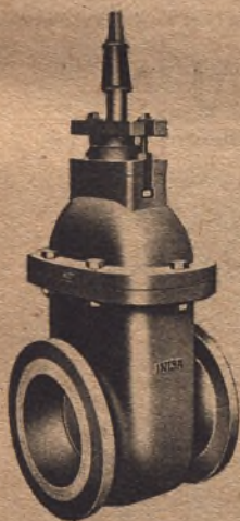
MODELO INGLES Paso nominal mm. 40 a 700 Presión trabajo Hasta 32 Kgs. cm. 2
