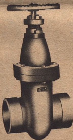
MODELO STANDARD Paso nominal mm. 50 a 250 Presión trabajo Hasta 16 Kgs. cm. 2
