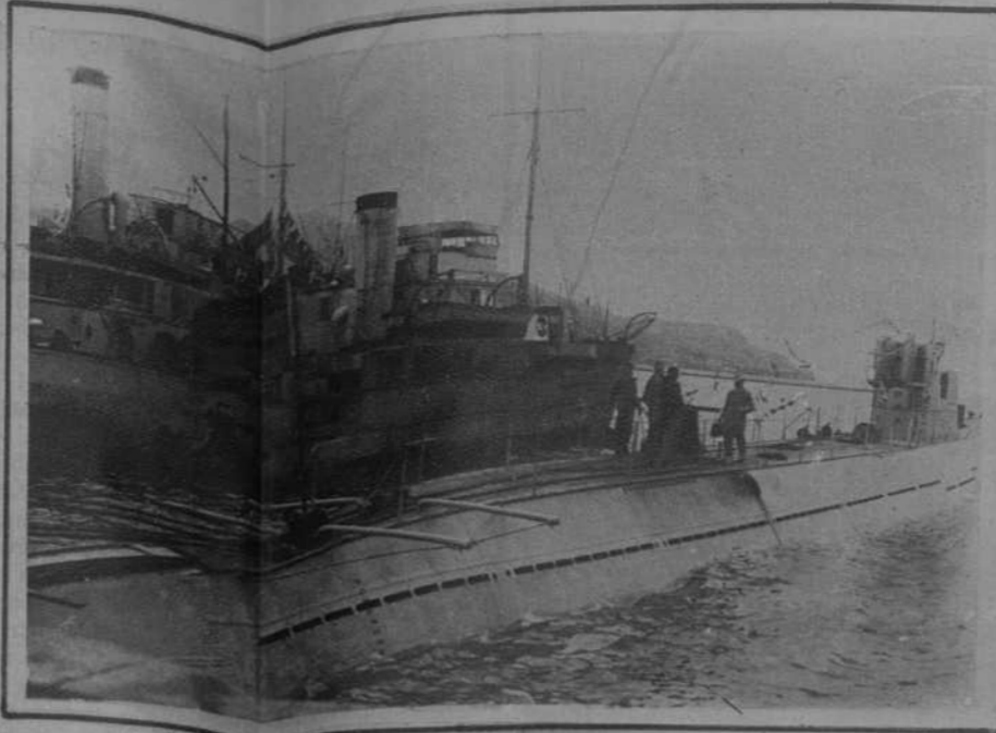
Cartagena.—Llegada del nuevo submarino «E. 1», construido en Cádiz, para realizar en este puerto pruebas de inmersión, a cien metros de profundidad. — (Fot. Izquierdo)
