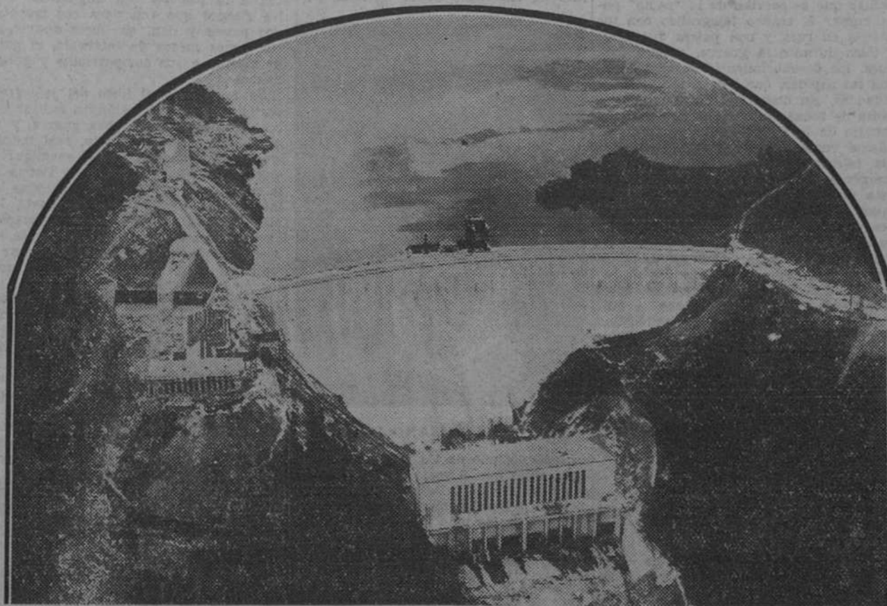
Dos años después. La presa de Bleiloch, con sus 180.000 metros cúbicos de hormigón, y su central de energía eléctrica abajo y su ferrocarril y sus construcciones accesorias, ya está completa.
