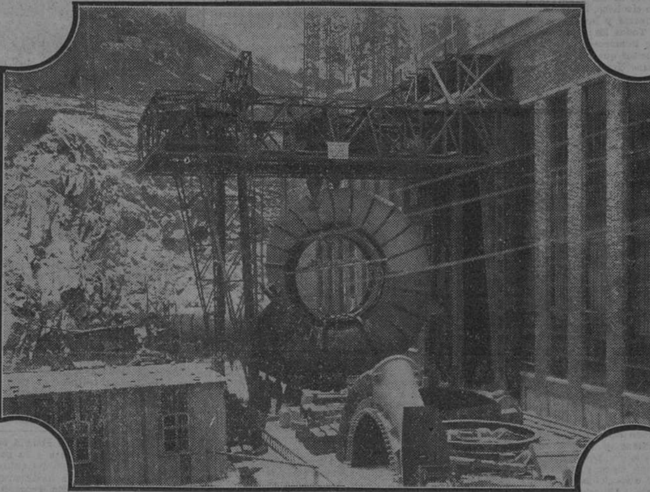
El caracol gigante de la turbina en marcha lenta y segura hacia su asiento, fuente de energía
