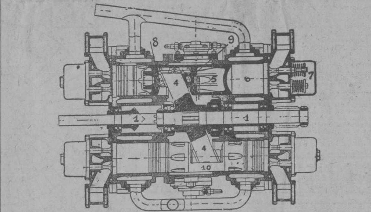
Esquema demostrativo del nuevo motor sin bielas inventado por el ingeniero australiano A. G. Mitchell...
