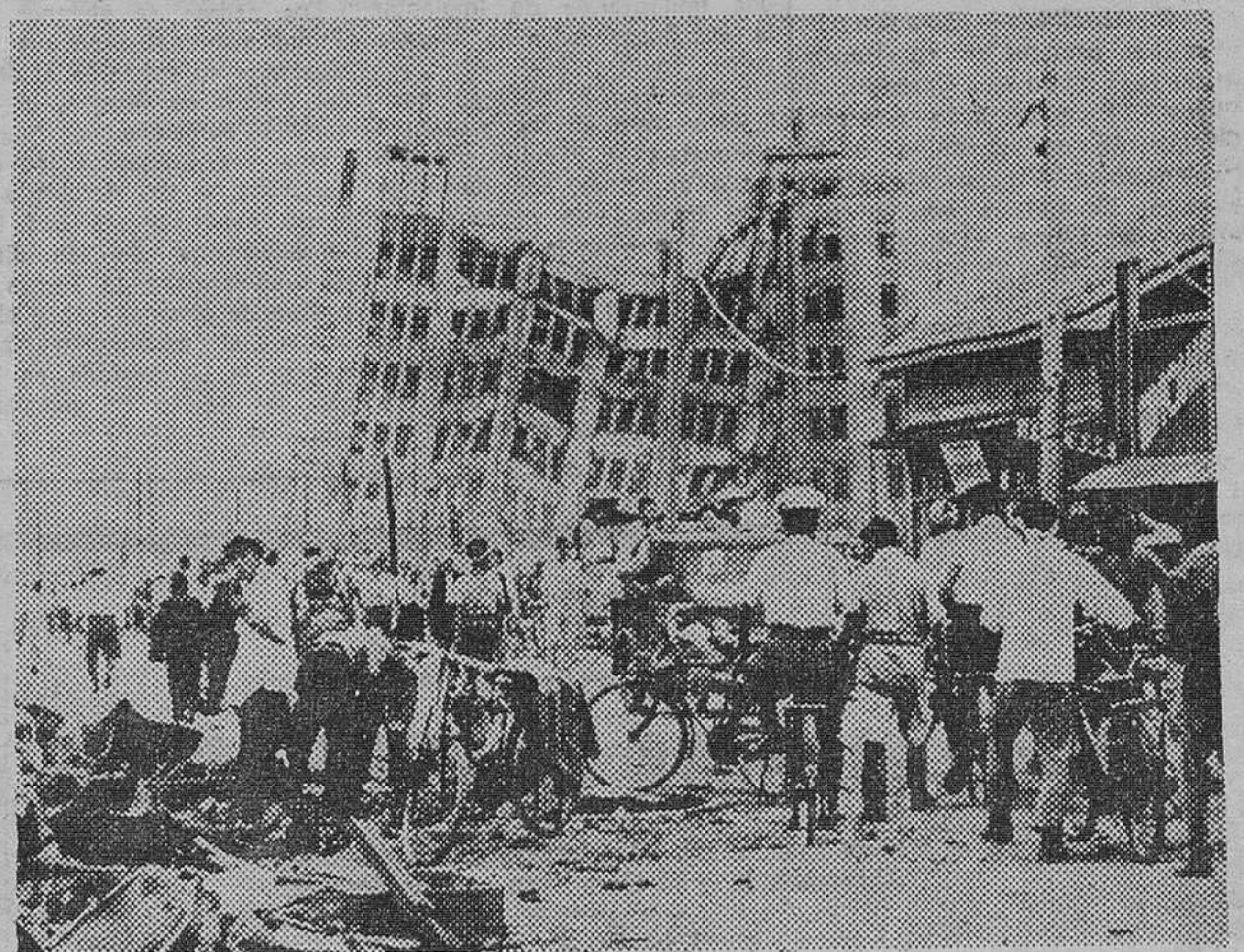
El archipiélago japonés se halla situado en una de las zonas geográficas de máxima sismicidad. He aquí el extraño aspecto de un edificio afectado en un reciente terremoto. — (Foto EFE-FIEL).
