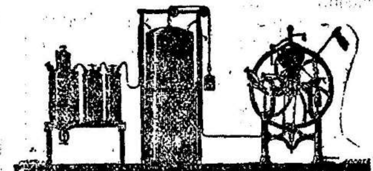
Aparatos para gaseosas, continuo, con embotelladoras unidas.
