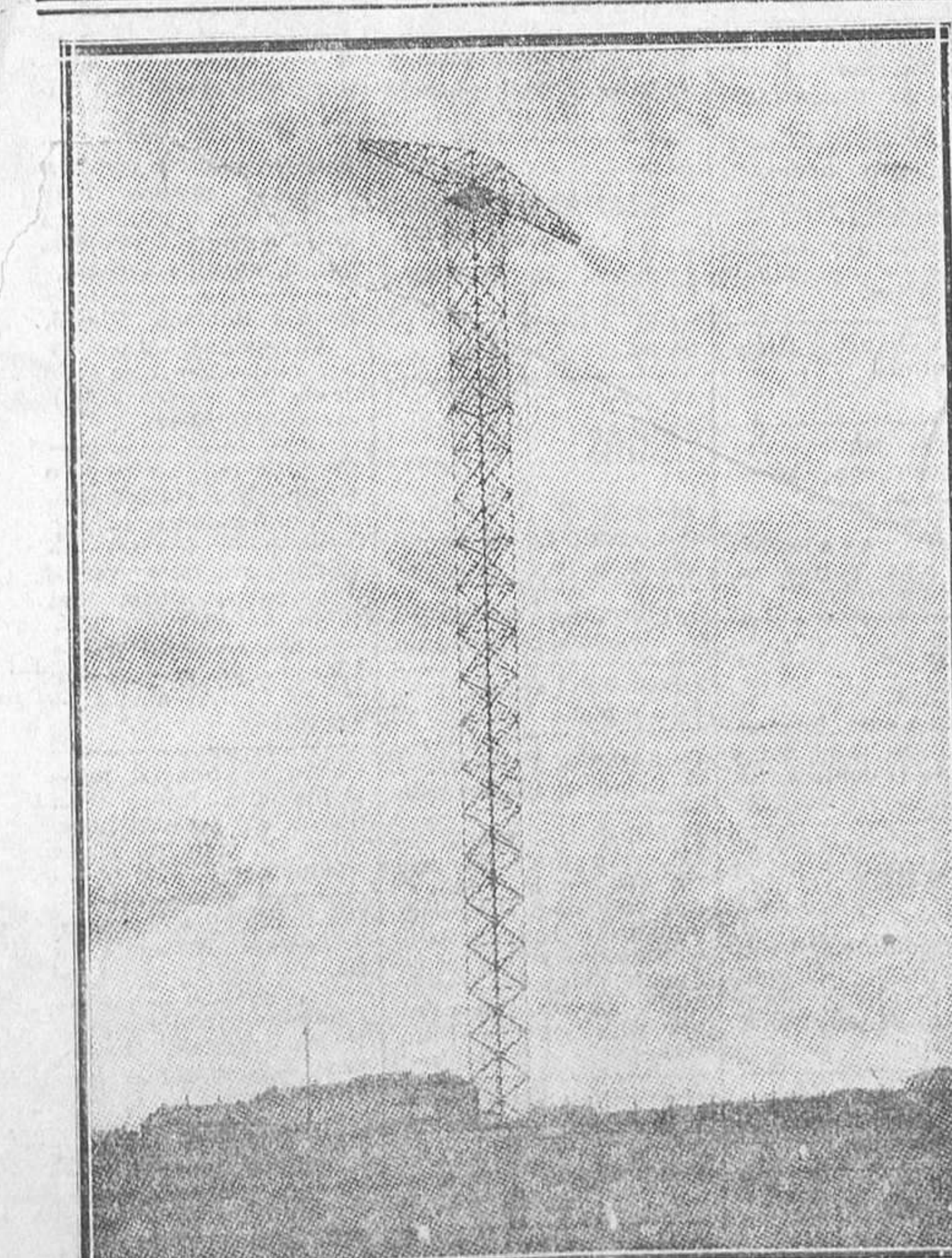
Una de las majestuosas torres de la emisora de Dorchester (Inglaterra), que comunica con las estaciones de la costa oriental de los Estados Unidos
