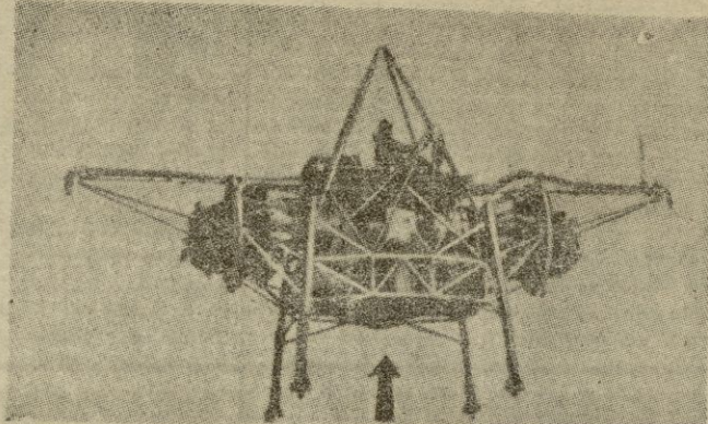
En la "cama volante", que despegue verticalmente, está inspirado el nuevo tipo de avión a reacción inventado por Stanley Kapelski
